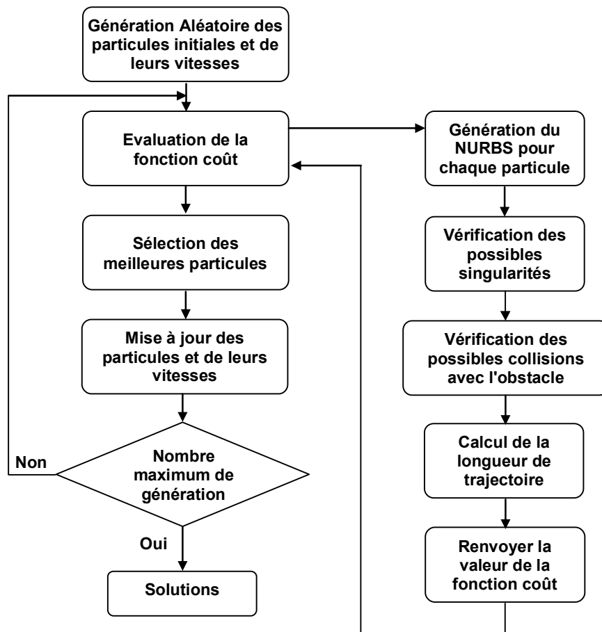
Figure 4.2 Organigramme de l'approche NURBS-Essais particulaires
