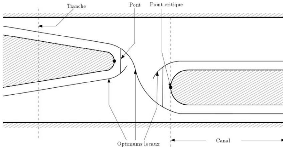
Figure 2.6. Planificateur de chemin opportuniste
