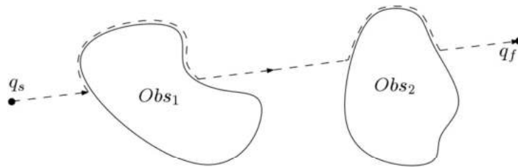
Figure 2.2. Planification des chemins par l'algorithme Bug2
