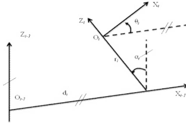
Figure 1.1. paramètres géométrique
