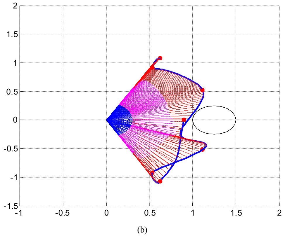
Figure 4.19. Trajectoire optimisée par les essaims particulaires dans un environnement avec un obstacle. (a) vue 3D. (b) vue 2D.
