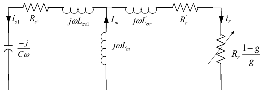
FIG. 2.2 – Schéma équivalent de l'auto-amorçage.
