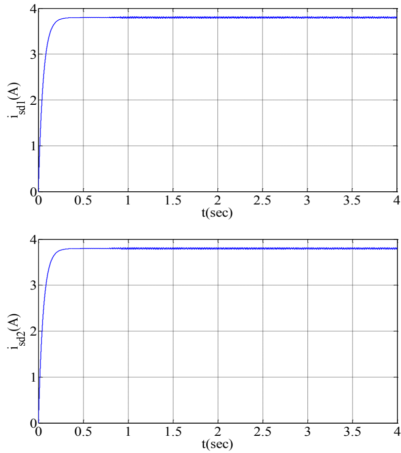
FIG. 4.8 – Courants i_{sd1} , i_{sd2} .
