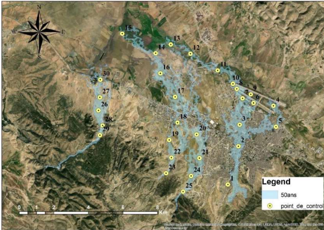
Figure 3.27 : La simulation de la crue 50 ans
