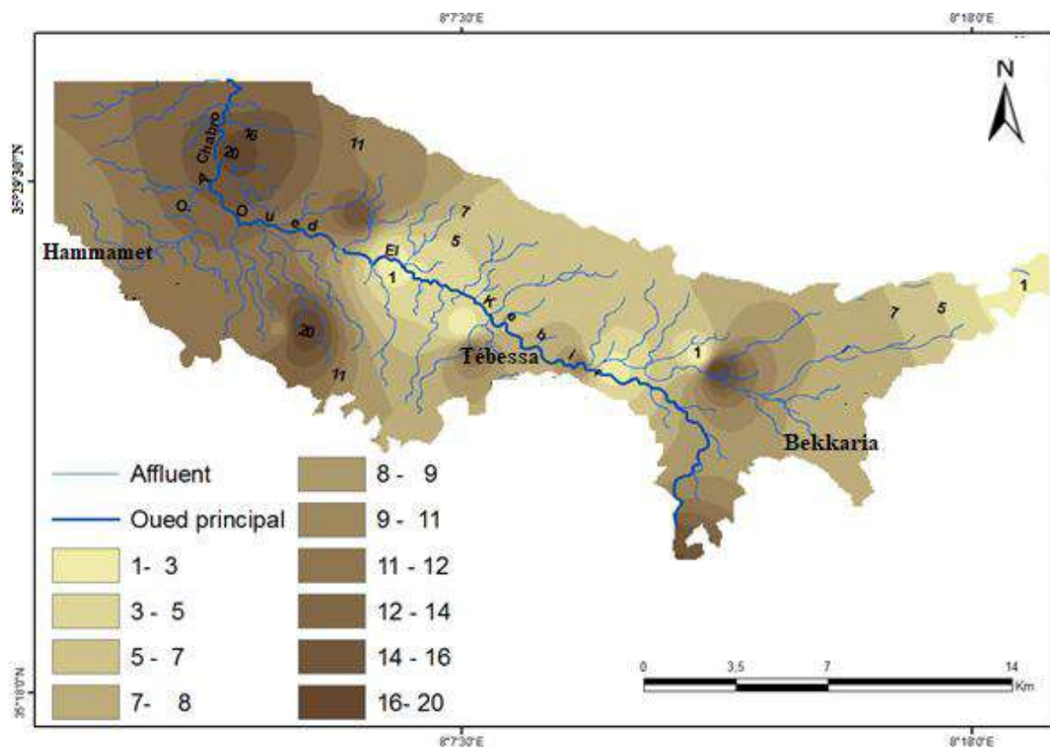
Figure 3.15: Carte d'isoteneurs en potassium (mg/l)
