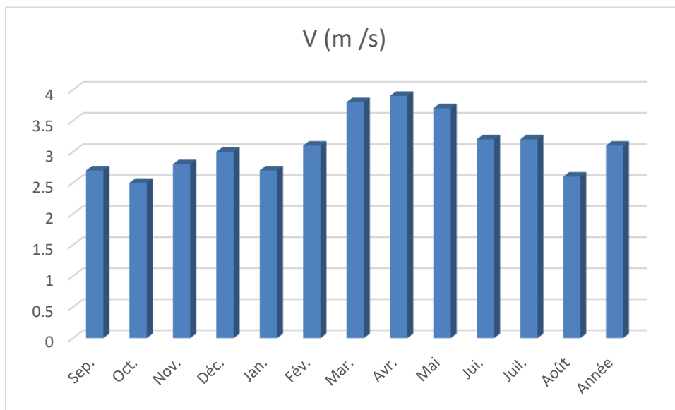
Figure 2.6 : Vitesse moyenne mensuelle du vent (m/s)
