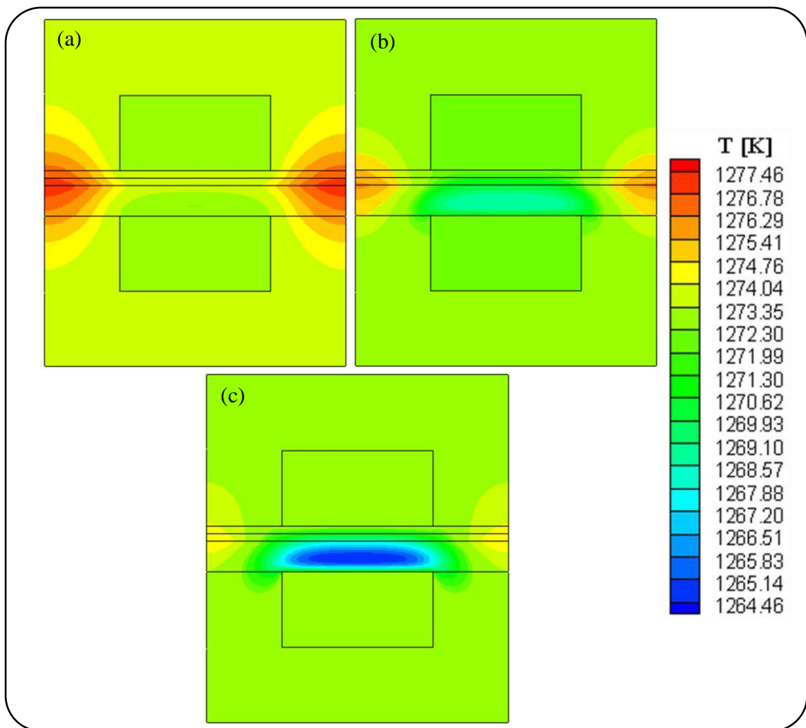
Fig. 4.14: Effet de la pression des gaz sur le champ thermique d'une pile SOFC en présence de la source de chaleur totale ( T_{\text{gaz}}=1273 [K]).
