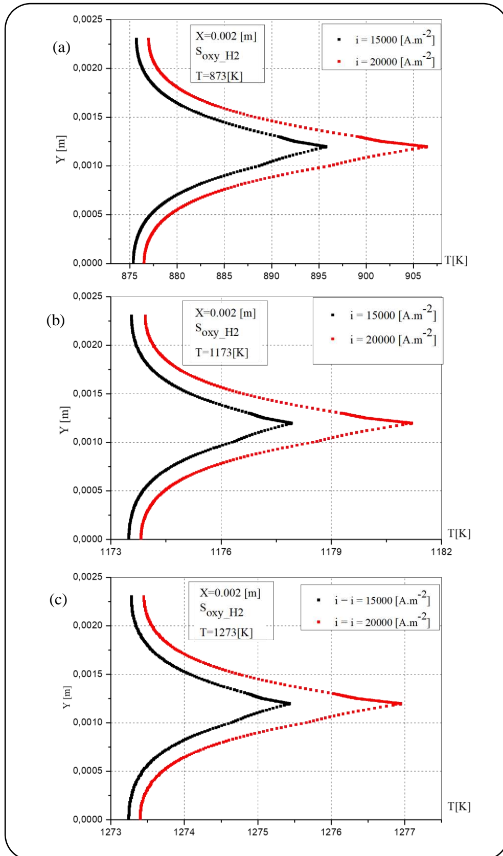
Fig. 4. 16: Effet de la densité de courant sur le profil de la température d'une pile SOFC en présence de la source de chaleur de la réaction d'oxydation de l'hydrogène ( S_{\text{ox}_y_{\text{H}_2}} ).
