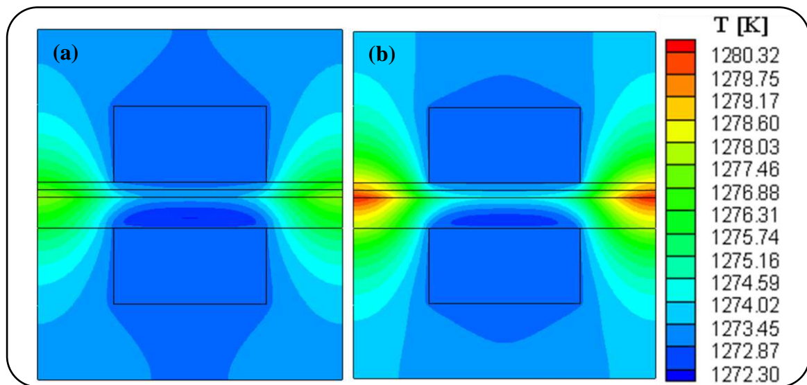
Fig. 4.20: Effet de la densité de courant sur les champs thermique d'une pile SOFC en présence de la source de chaleur totale ( T_{\text{gaz}}=1273 [K]). (a): i = 15000 [ \text{A.m}^{-2} ], (b): i = 20000 [ \text{A.m}^{-2} ].
