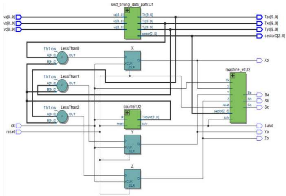
Figure.III.17 Schéma RTL de la SVPWM optimisée.
