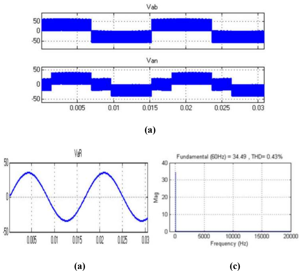
Figure II.22. Résultats de simulation de THIPWM, a). Tension de sortie de l'onduleur composé et simple, b). Tension simple filtrée, c). Spectres de la tension filtrée.
