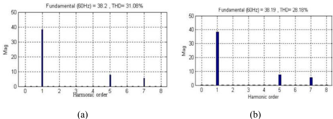
Figure II.16. (a): Spectre harmonique de la tension simple Van, (b): Spectre harmonique de la tension de sortie du filtre V1R
