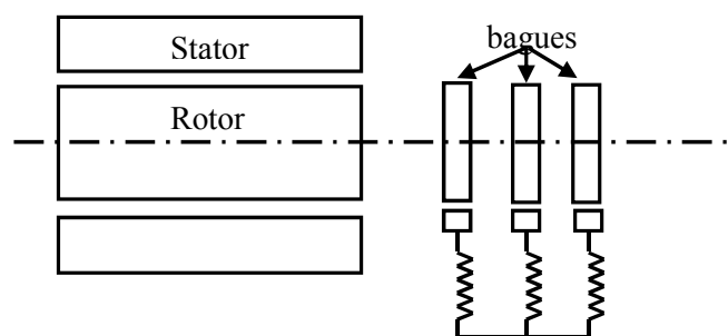
Figure I.1 Principe du rotor bobiné
