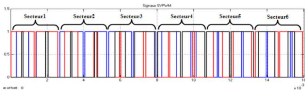
Figure II.23. Allure des signaux SVPWM générés à f=60\text{Hz} , f_c=12*f , m=0.9
