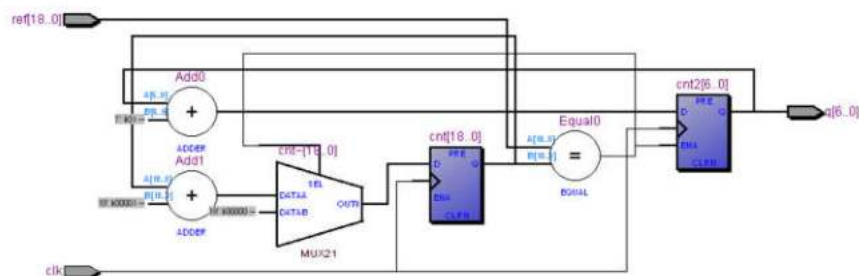
Figure.III.6 vu niveau RTL du compteur pointeur.
