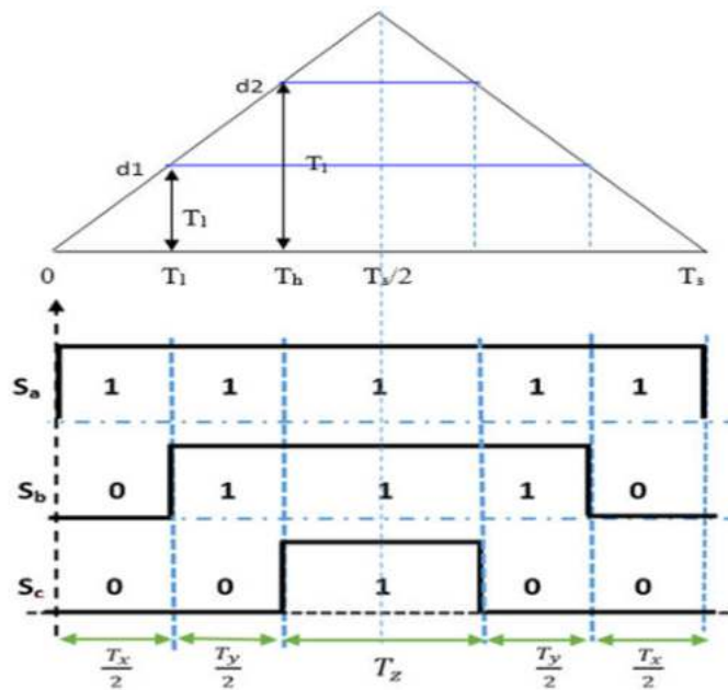
Figure III.16 génération des signaux de commande
