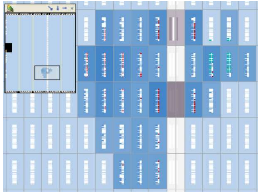
Figure III.14 Occupation physiques, sur FPGA, des différents Blocs Logiques implémentant le THIPWM.
