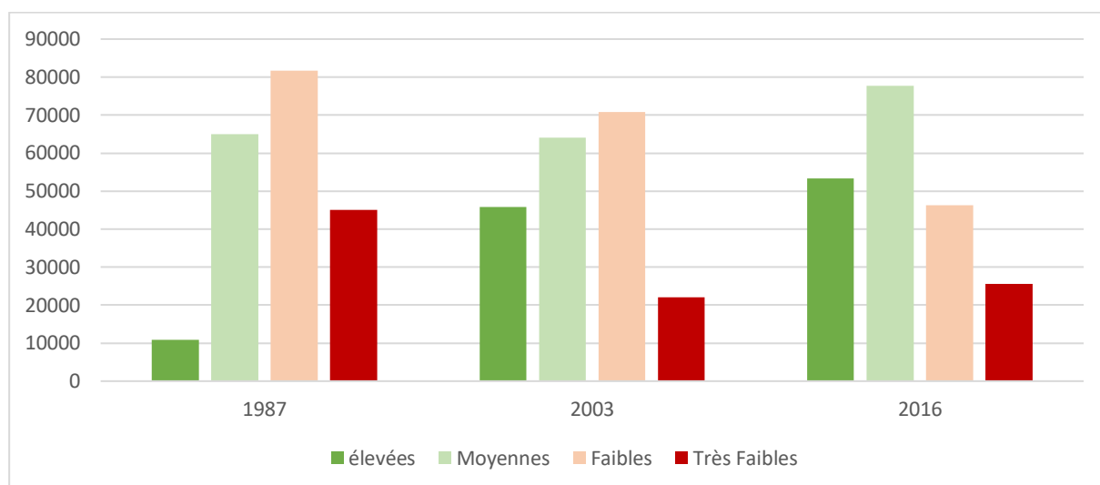
Figure 51 : La superficie des classes de l'NDVI par hectare pour les années 1987, 2003, 2016.
