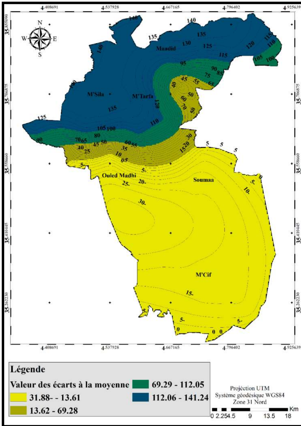
Figure 39 : Carte des écarts à la moyenne.
