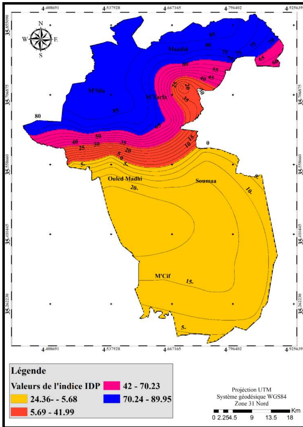
Figure 36 : Carte de l'indice de déficit hydrique de la zone d'étude.
