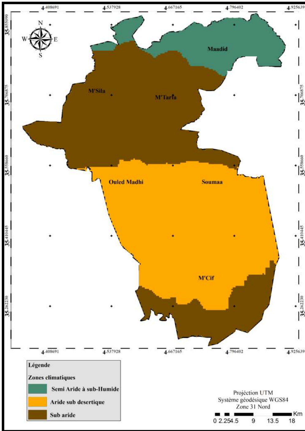
Figure 18 : Carte de zones climatiques (Sebhi, 1987)
