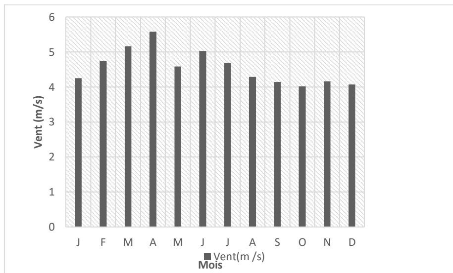
Figure 28 : Histogramme des moyennes mensuelles et annuelles de la vitesse du vent en (m/s) de la région de M'Sila (1988-2016)
