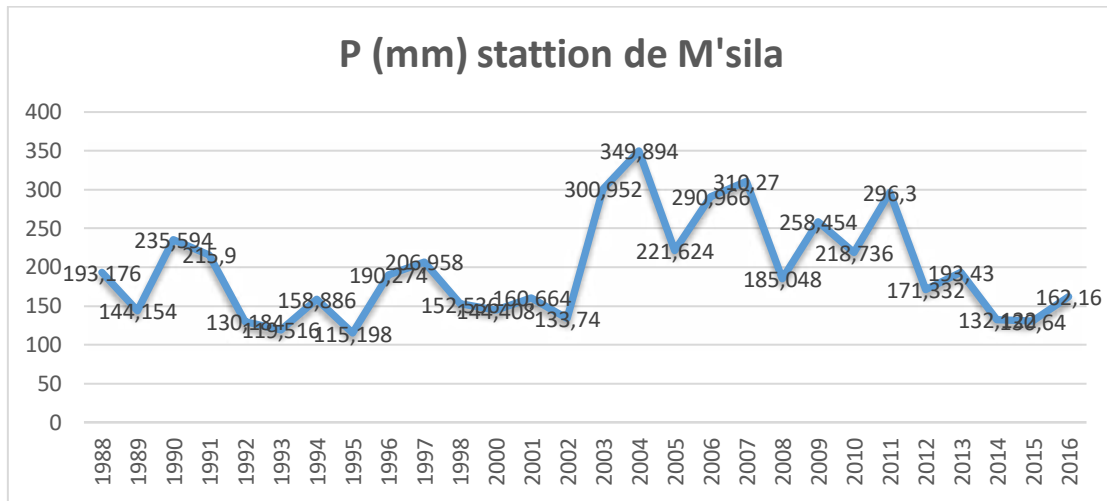
Figure 19. Fluctuations des taux de précipitations annuelles de la station de M'sila (1988 – 2016)
