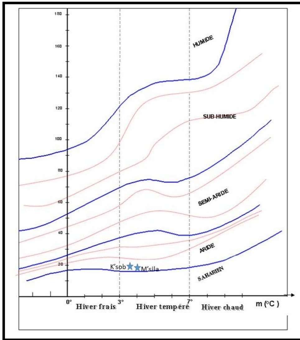
Figure 33 : Diagramme pluviothermique de la zone d'étude
