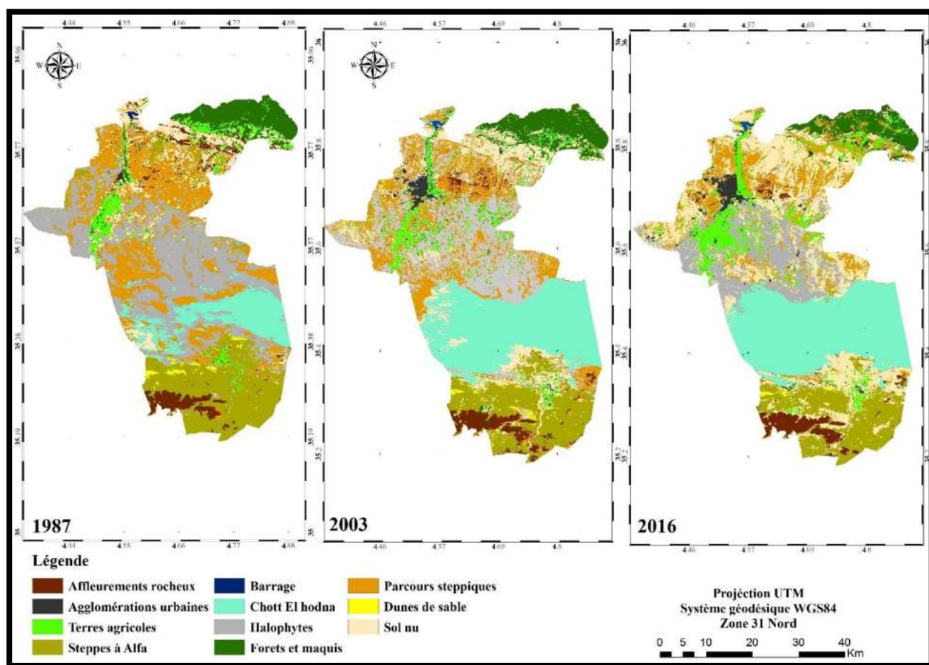
Figure 45 : Cartes d'occupation du sol en 1987- 2003- 2016
