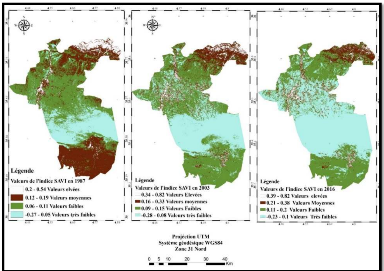
Figure 57 : Cartes de l'indice ajusté de sol et de végétation
