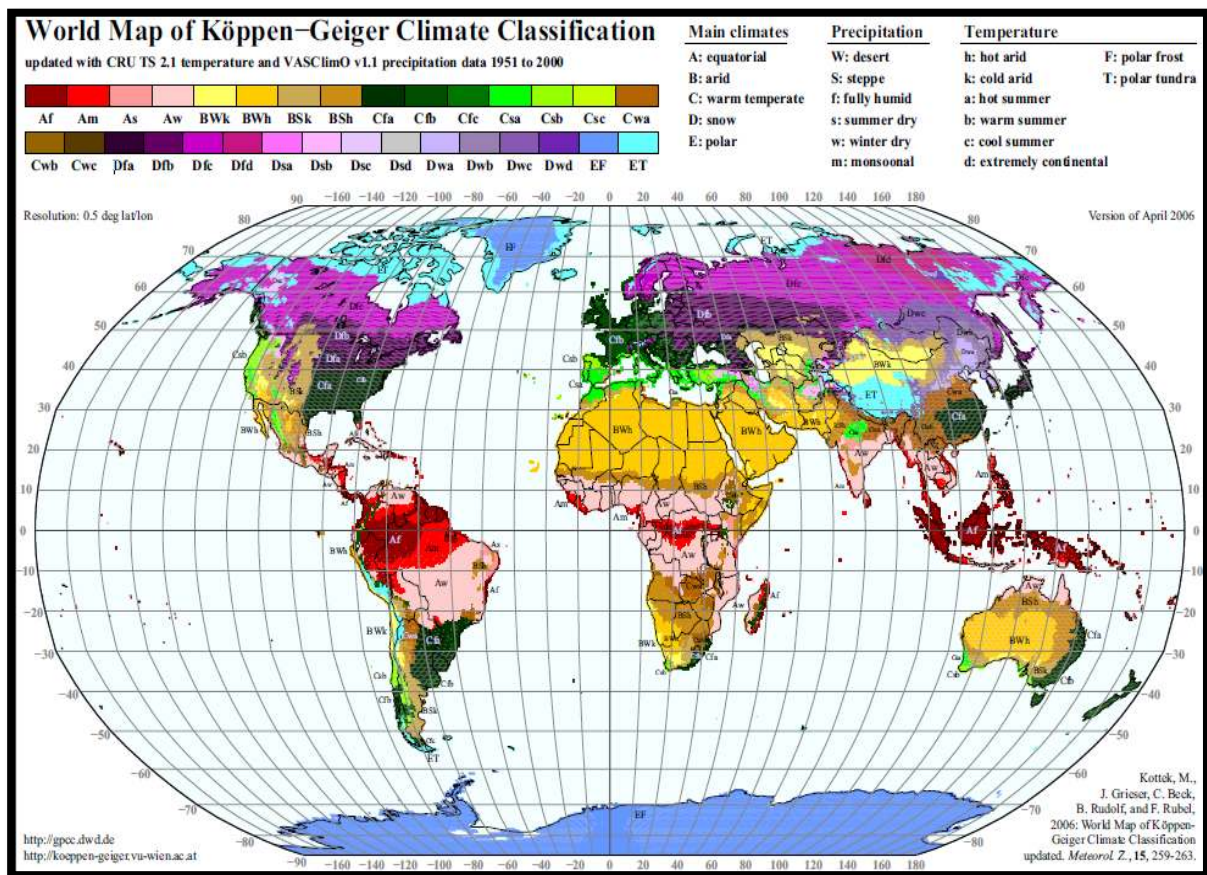
Figure 40: La carte mondiale de classification de Köppen- Kreiger, Carte mise à jour, (Kotték ., et al, 2006).
