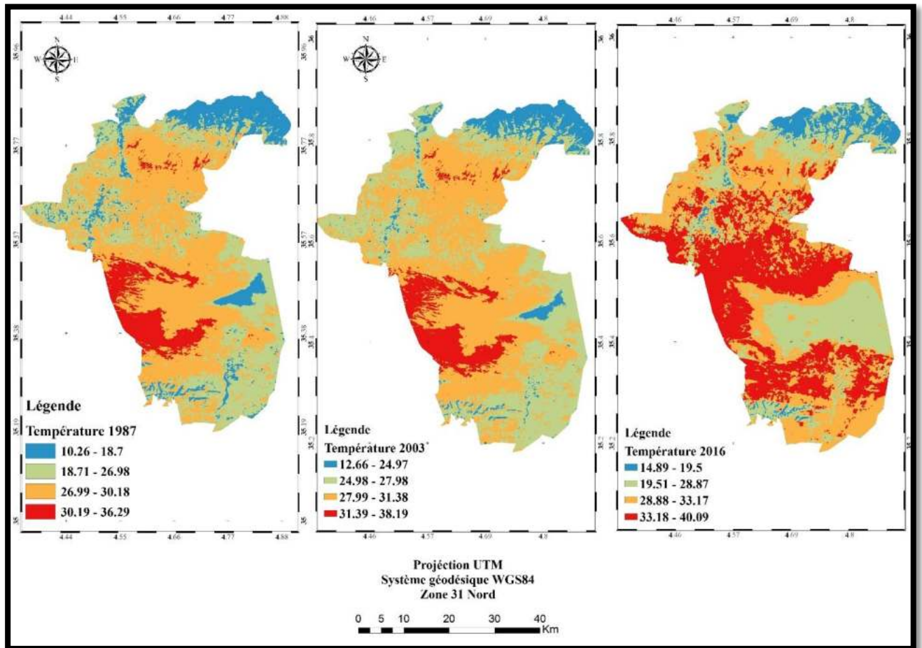
Figure 59 : Carte de la température de la surface du sol estimée dans l'année 1987, 2003,2016.
