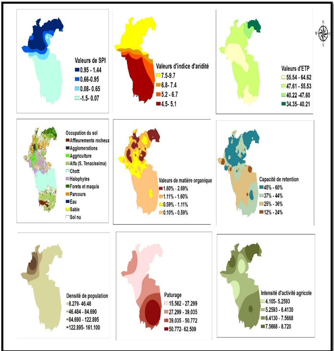
Figure 62 : Carte des sous-critères
