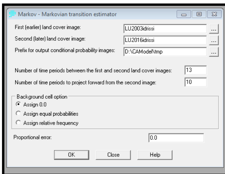
Figure 79 : Création de transition d'estimation MARKOV
