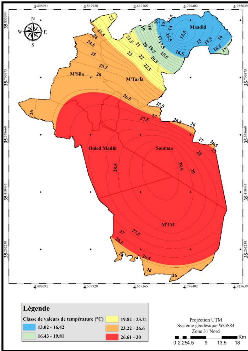
Figure 27 : Distribution spatiale des températures moyennes
