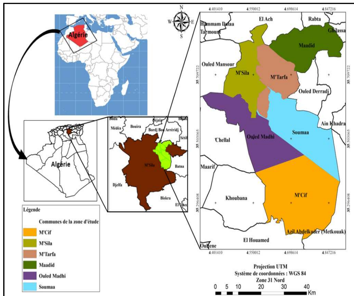
Figure 1: Situation géographique de la zone d'étude
