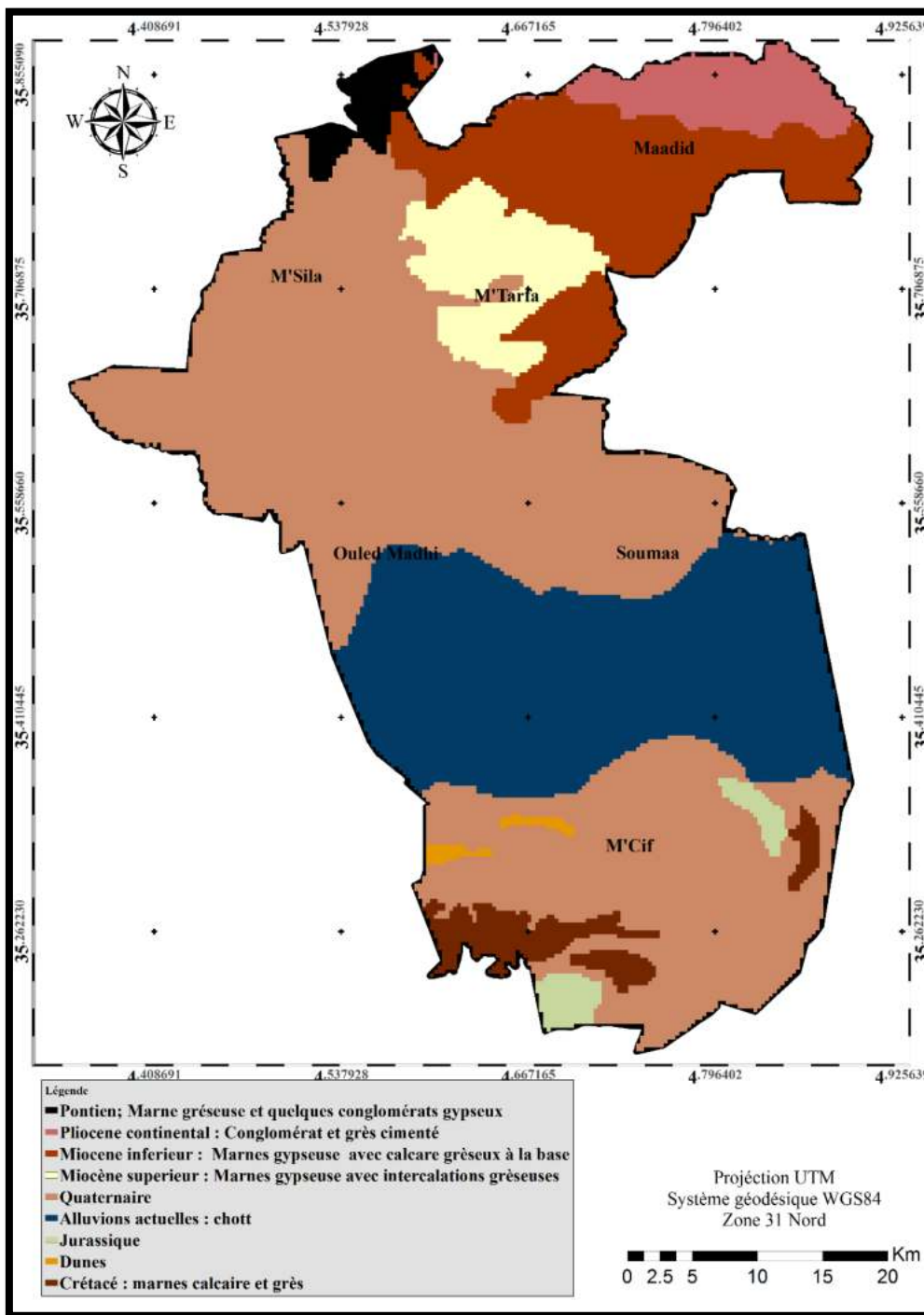
Figure 5 : Carte géologique de la zone d'étude (extraite de la carte de Amroun, 2008)
