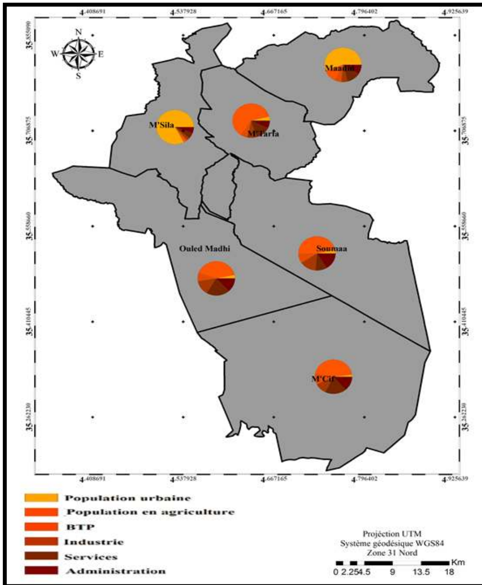
Figure 13 : Occupations de population de la zone d'étude (Source : Conservation des forêts de la wilaya de M'sila : Monographie des commune 2014/2015)
