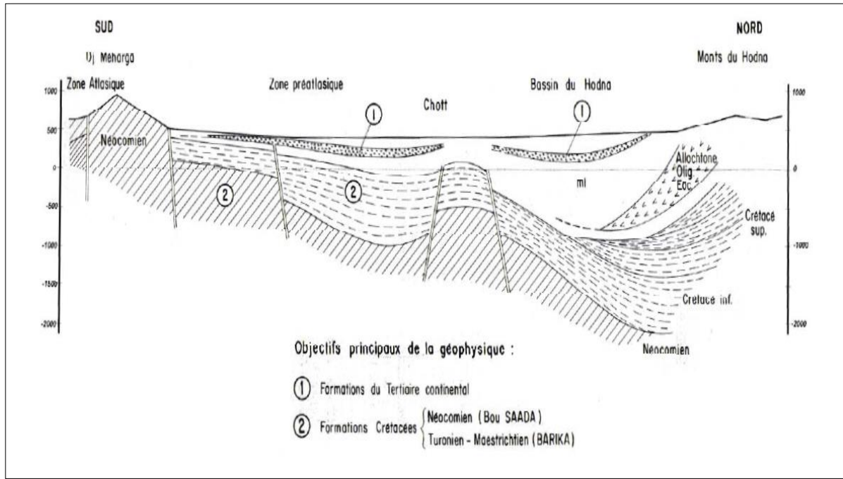
Figure 6 : Coupe géologique de l'avant pays de la chaîne alpine en Algérie, au niveau du Hodna oriental (Guiraud, 1971)
