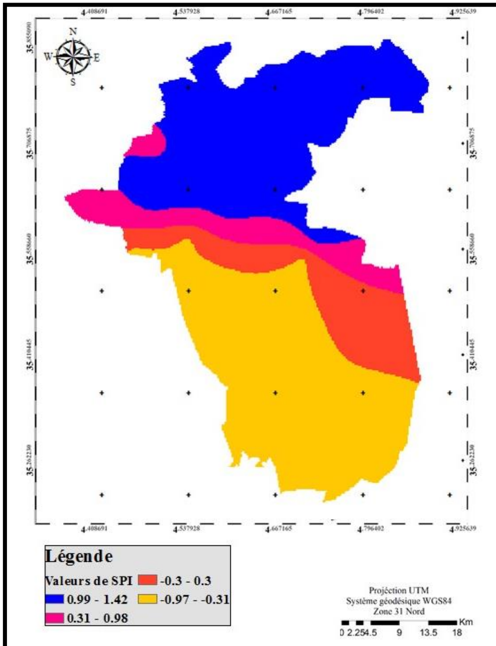
Figure 37 : Carte de l'indice SPI de la zone d'étude de l'année 2016
