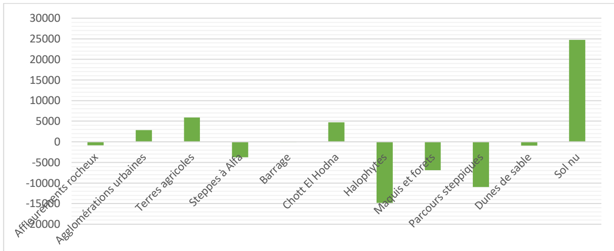
Figure 47 : Différence entre les surfaces d'occupation du sol entre 2003-2016 en hectare.
