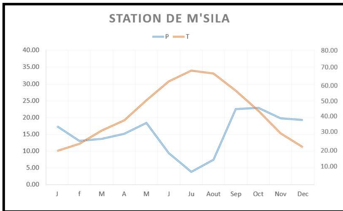
Figure 31 : Diagramme ombro-thermique de la station de M'Sila (1988-2016).
