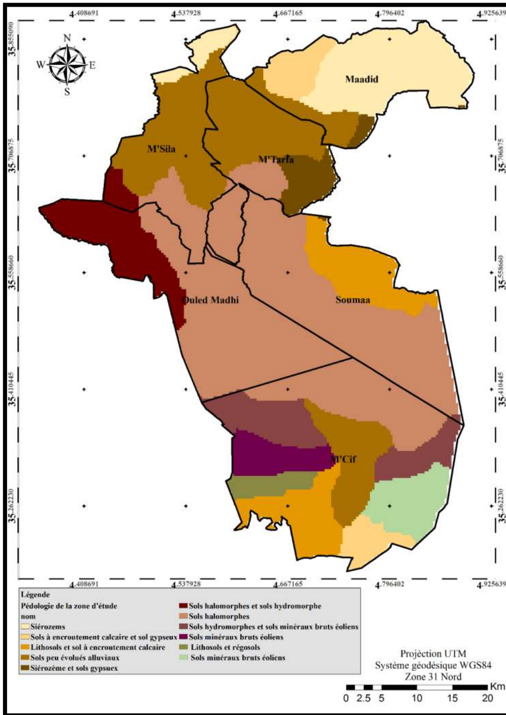
Figure 8 : Carte pédologique de la zone d'étude (Source : F.A.O, 1975).
