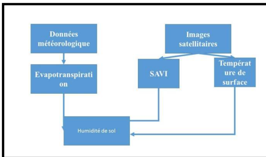
Figure 69 : Modèle conceptuel pour le calcul de l'humidité du sol (Cissoko, 2011).
