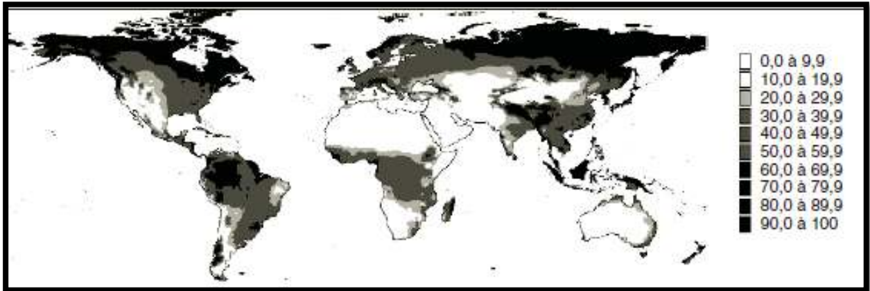
Figure 41: Zones caractérisées par leur valeur de l'indice d'aridité de Martonne, calculé pour la période 1951-2000
