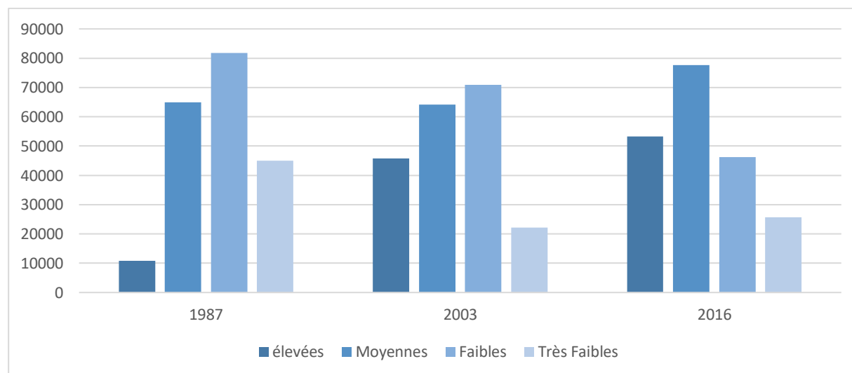
Figure 55 : La superficie des classes de l'indice de salinité par hectare pour les années 1987, 2003, 2016
