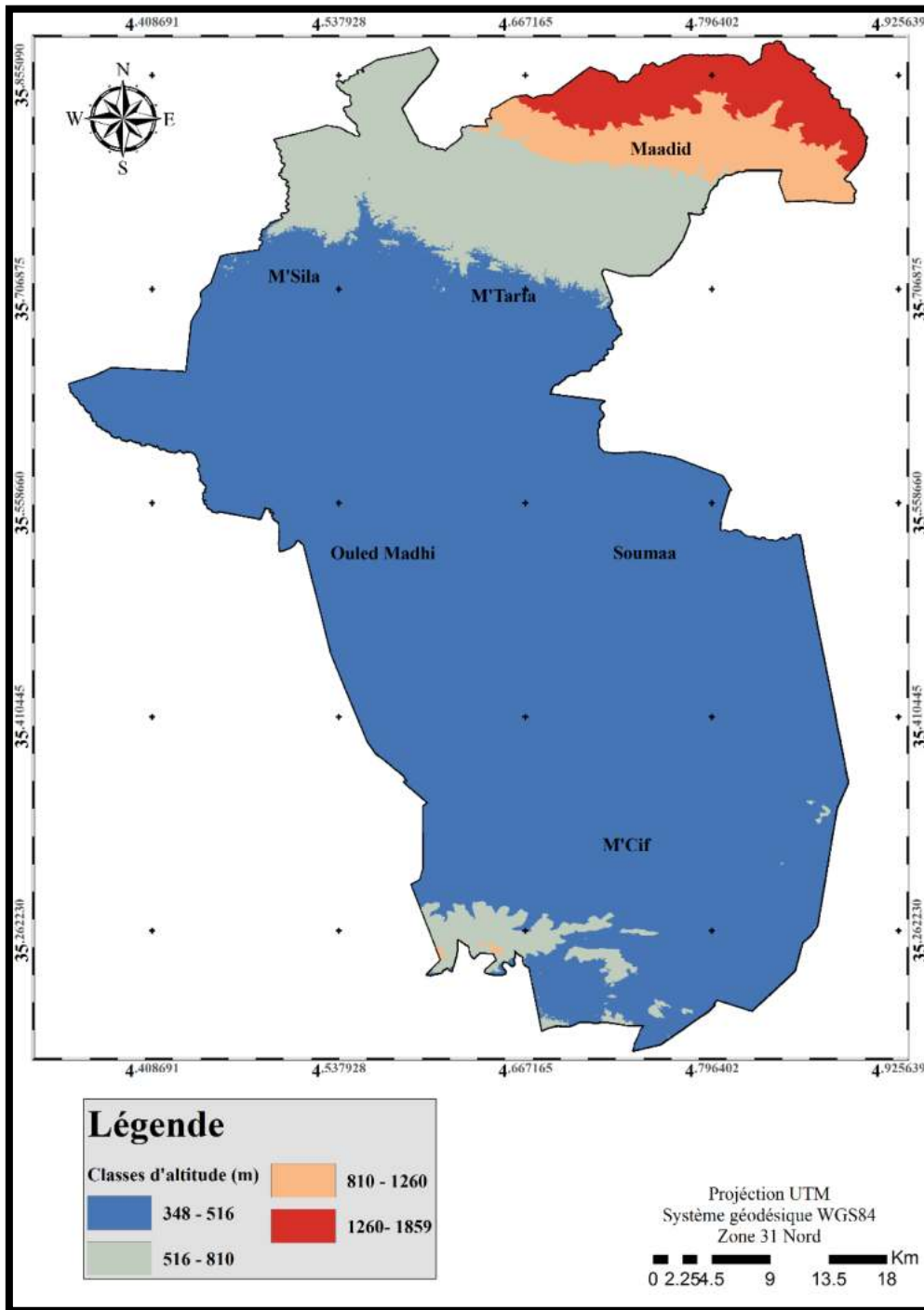
Figure 3 : Carte d'altitude de la zone d'étude (extraite du modèle numérique du terrain MNT)
