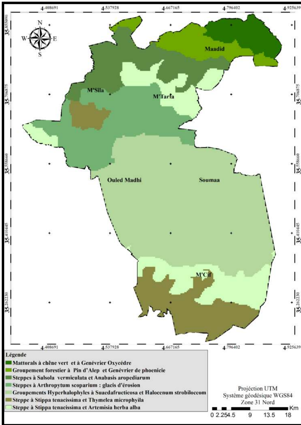
Figure 11 : Carte Phyto-écologique de la zone d'étude (Source : Claudin et al., 1975)
