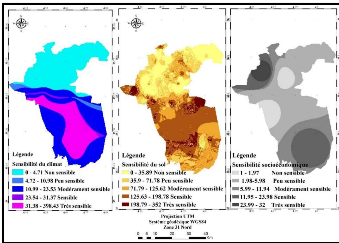
Figure 64 : Cartes de sensibilité climatique-édaphique- socioéconomique zones d'étude
