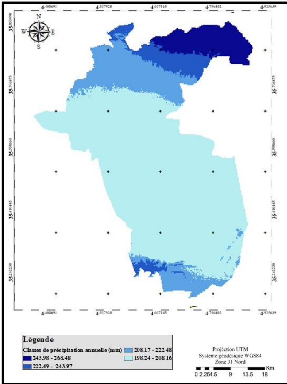
Figure 21 : Distribution spatiale des précipitations de la zone d'étude
