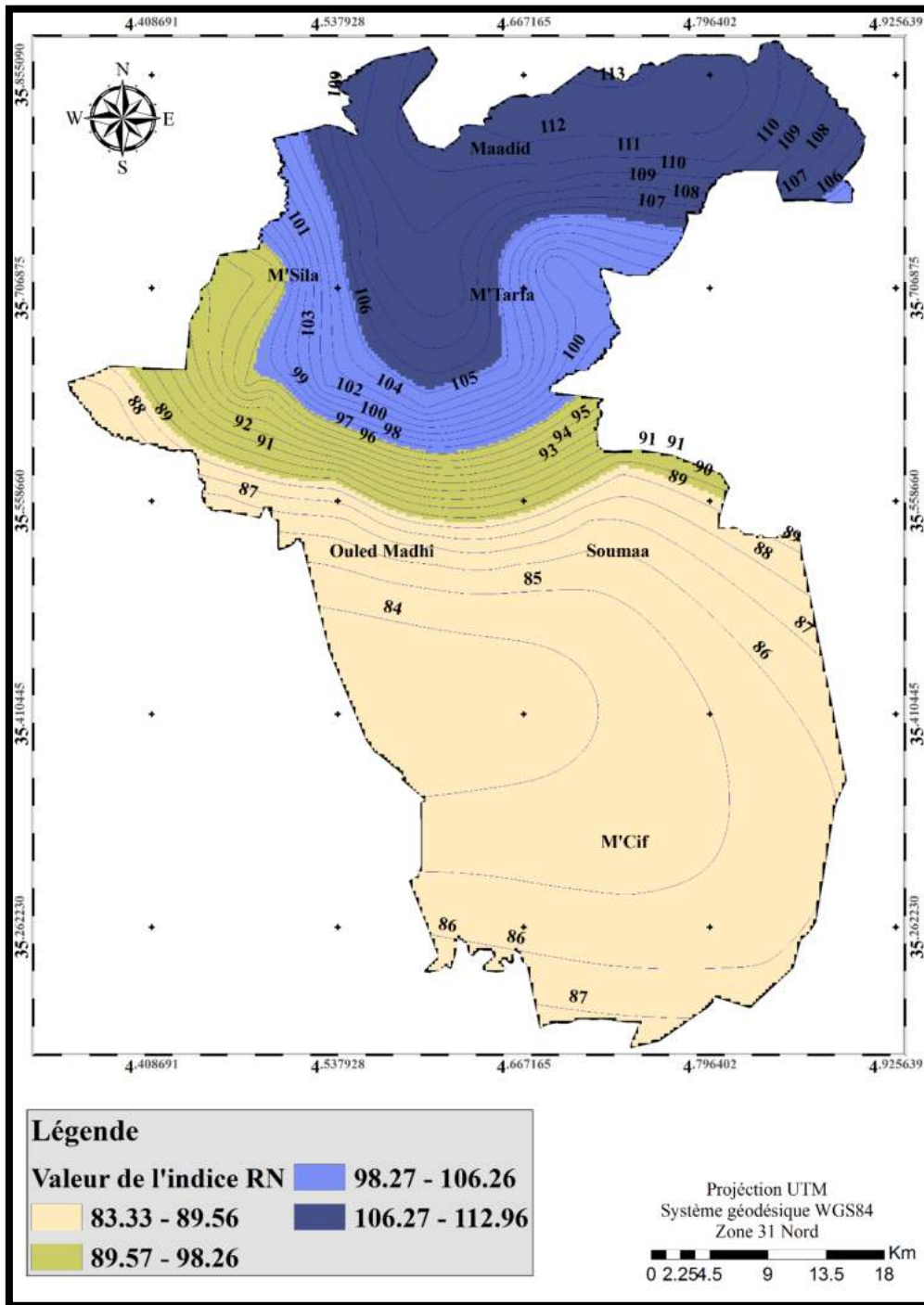
Figure 38 : Carte de l'indice rapport à la normal
