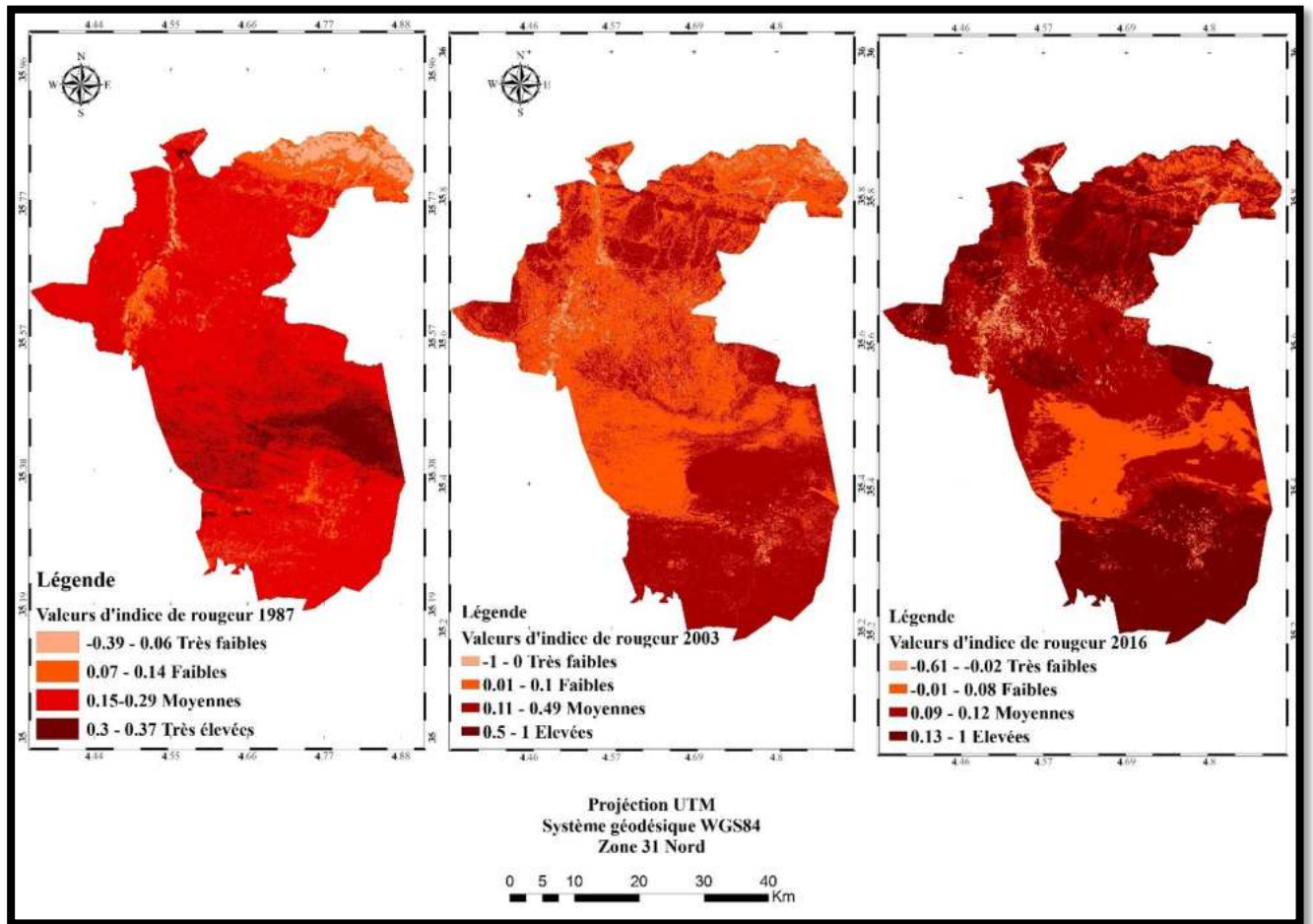
Figure 52 : carte de l'indice de rougeur (IR) (1987, 2003, 2016)
