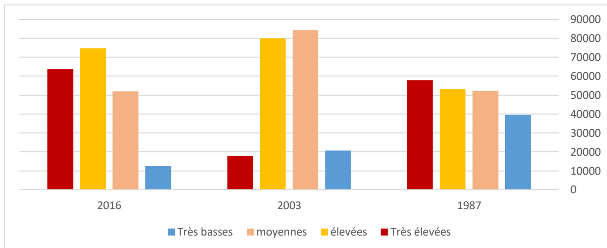
Figure 60 : La superficie des classes de la température de la surface du sol par hectare pour les années 1987, 2003, 2016
