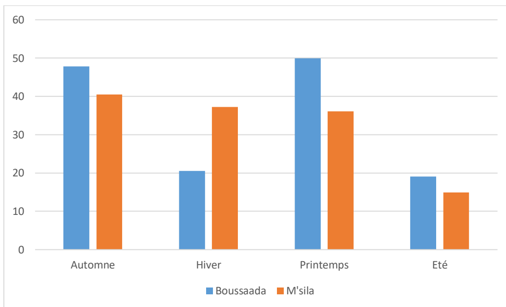
Figure 22 : Histogramme du régime saisonnier des stations de la région d'étude
