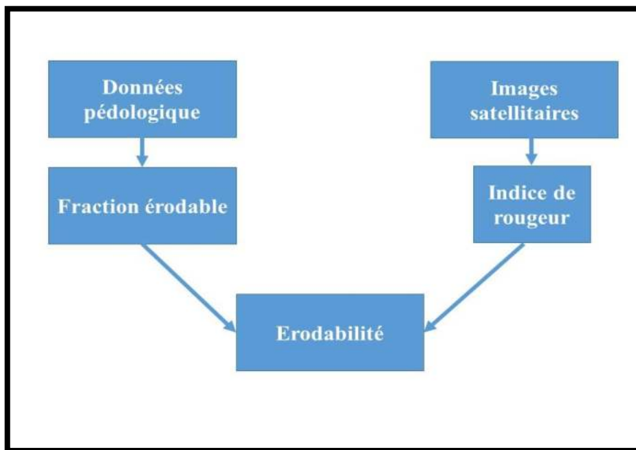
Figure 68 : Modèle conceptuel pour le calcul de l'érodabilité (Cissoko, 2011)
