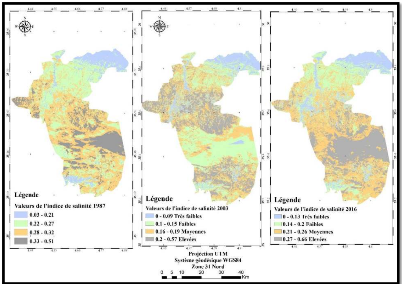
Figure 54 : Carte d'indice de salinité (2016, 2003, 1987)
