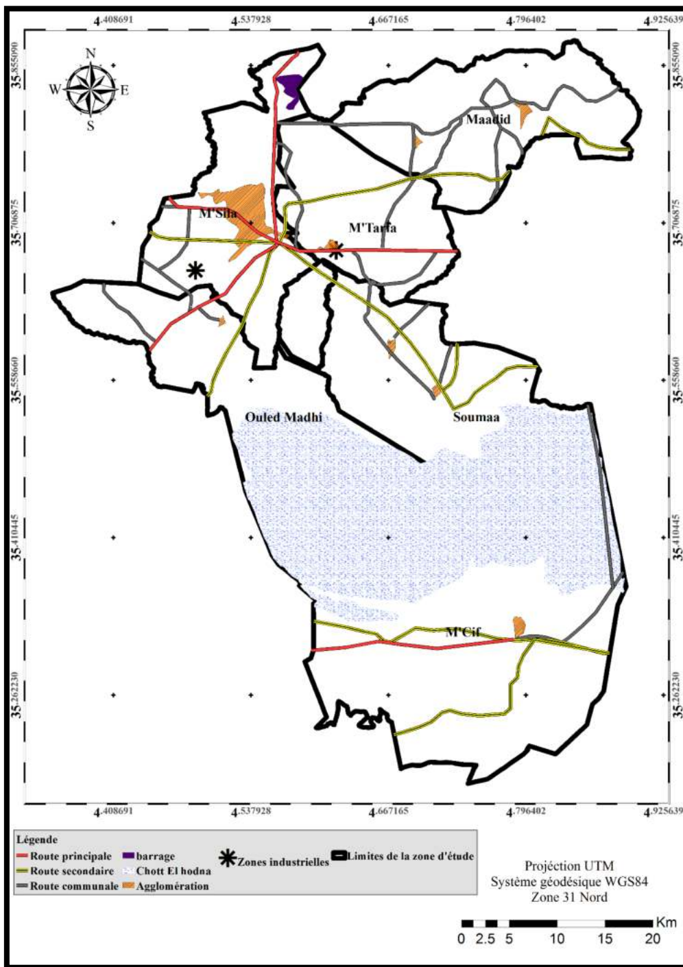
Figure 17 : Carte du réseau routier de la zone d'étude
