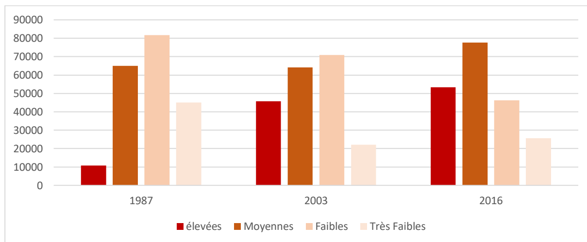
Figure 53 : La superficie des classes de l'indice de rougeur par hectare pour les années 1987, 2003, 2016
