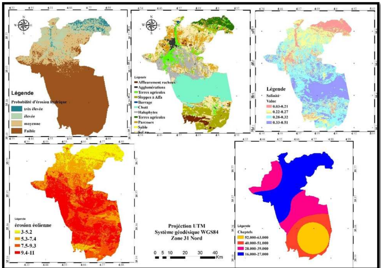
Figure 71 : Critères entrants dans la cartographie de la vulnérabilité à la désertification.
