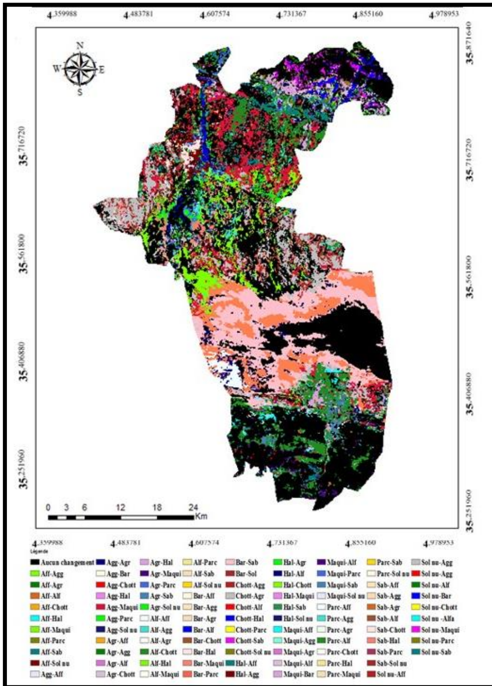
Figure 49 : Carte des unités de changements d'occupation du sol entre 1987 et 2016
