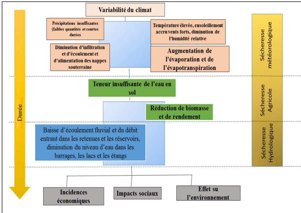
Figure 42: Succession et incidences des types de sécheresse
