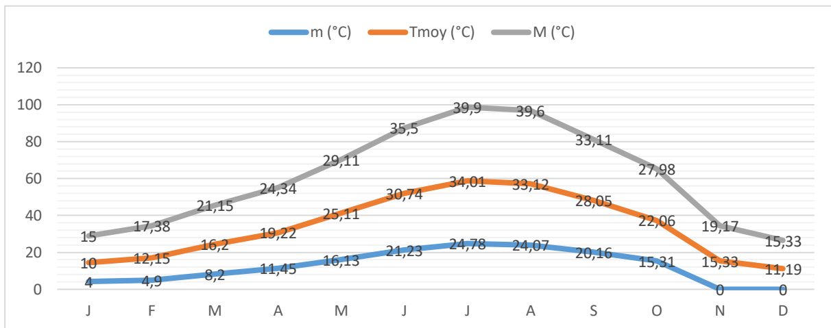
Figure 24 : Les courbes des températures minimales, moyennes et maximales mensuelles et annuelles (°C) de la région de El K'sob.
