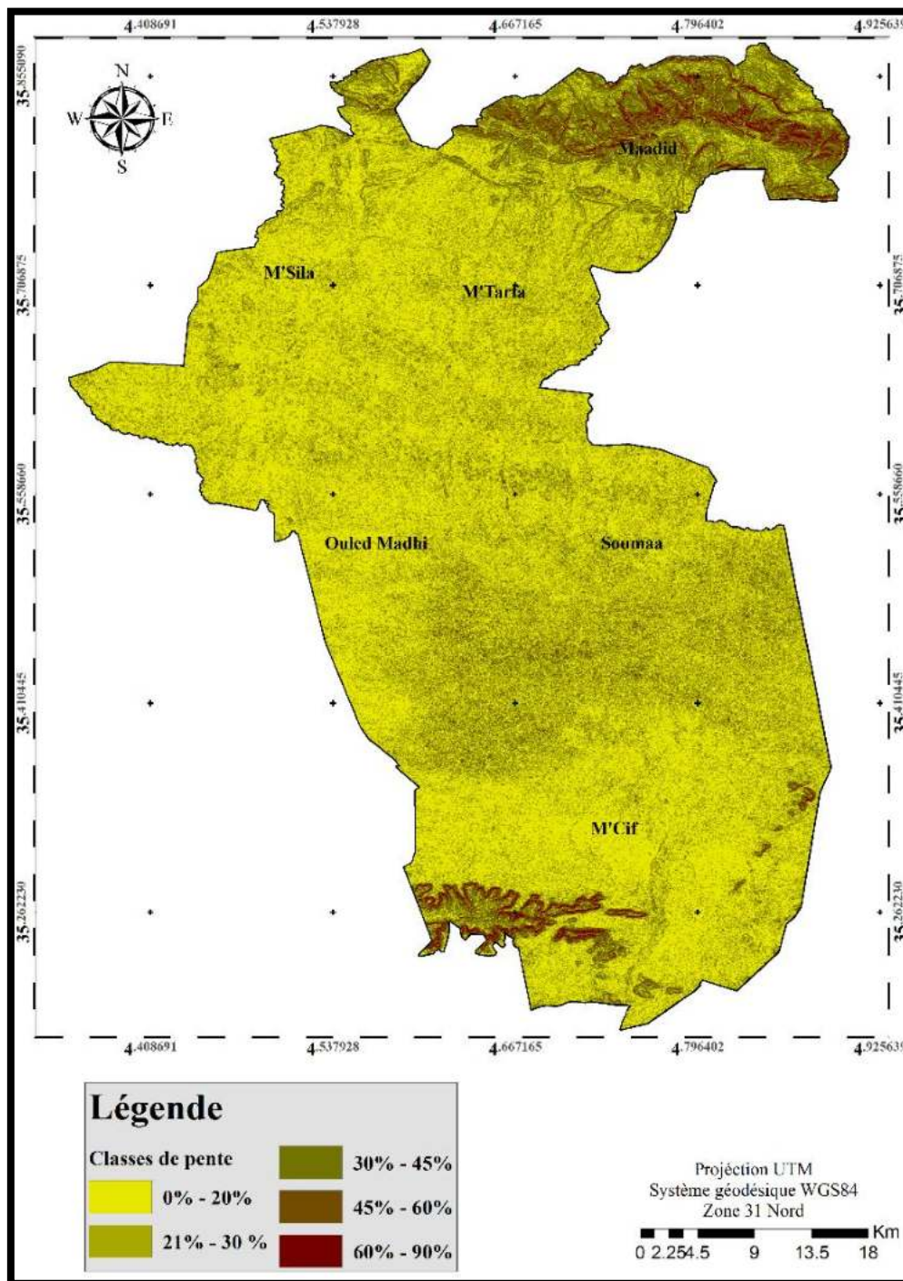
Figure 4 : Carte des pentes de la zone d'étude (extraite du modèle numérique du terrain MNT)
