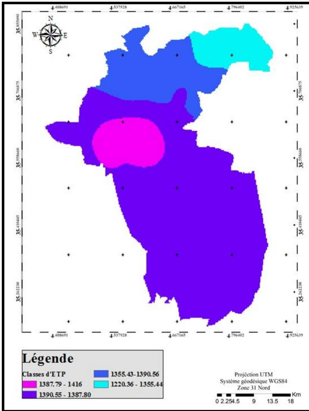
Figure 29 : Carte des valeurs d'évapotranspiration potentielle (en mm).
