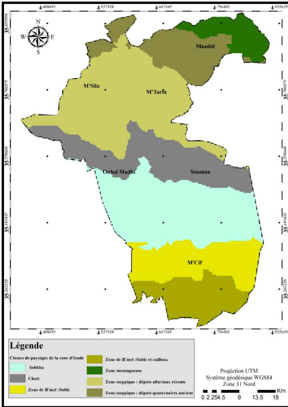
Figure 2 : Carte des paysages de la zone d'étude (Sebhi,1987)
