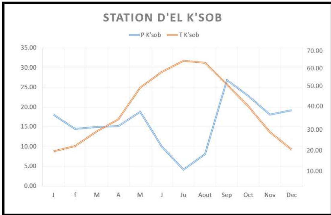
Figure 32 : Diagramme ombro-thermique de la station d'El K'sob (1988-2016).
