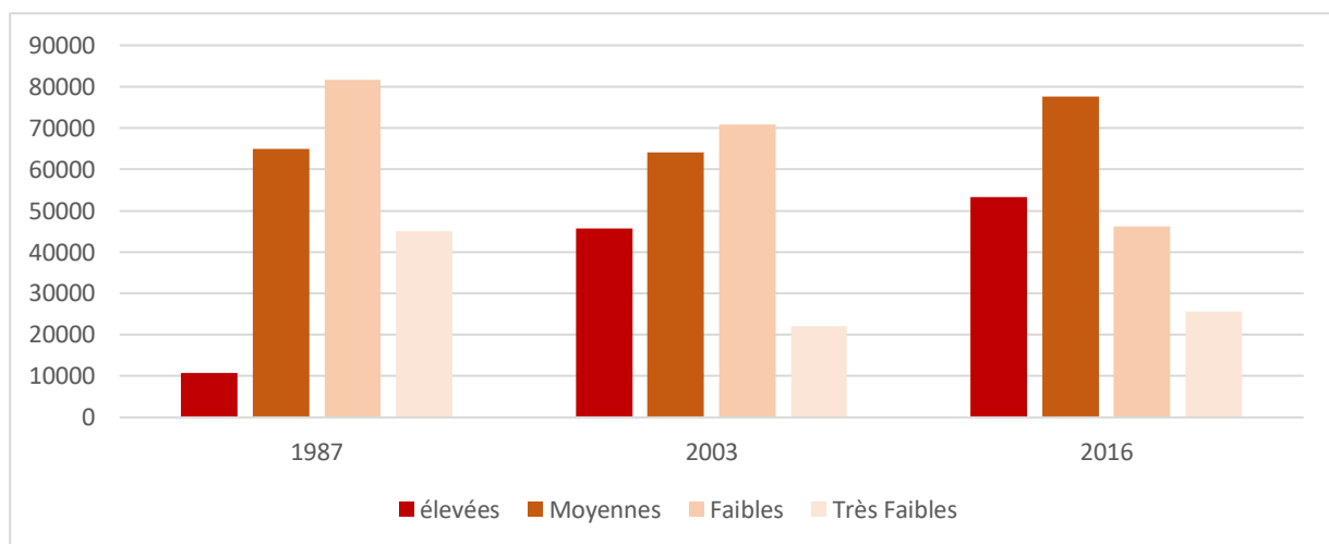
Figure 58: La superficie des classes de l'indice SAVI par hectare pour les années 1987, 2003, 2016
