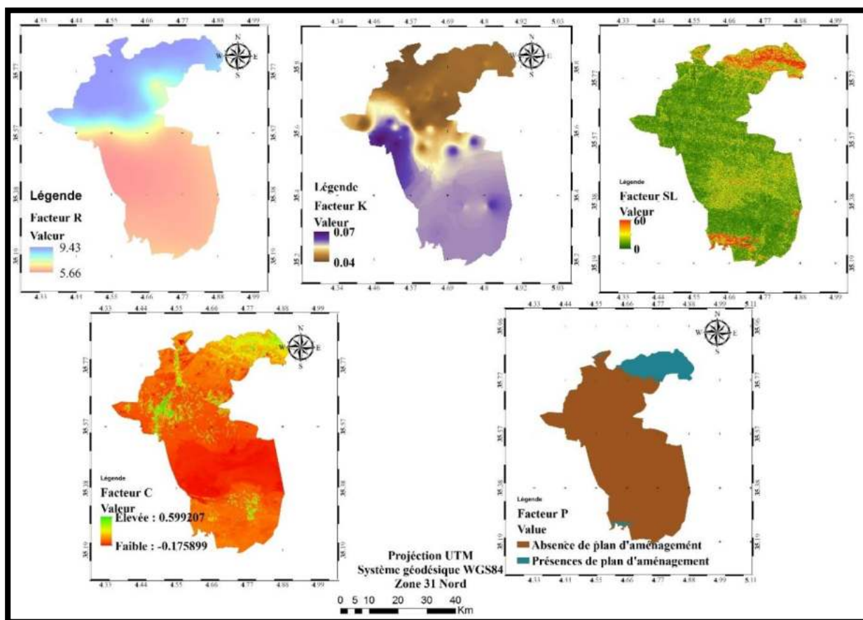
Figure 67 : Cartographie des facteurs entrés dans le calcul de l'équation de perte de sol USLE.
