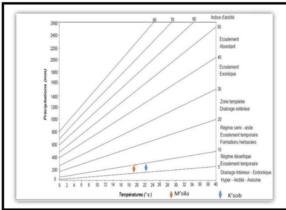
Figure 35 : Abaque de l'indice d'aridité de Demarton
