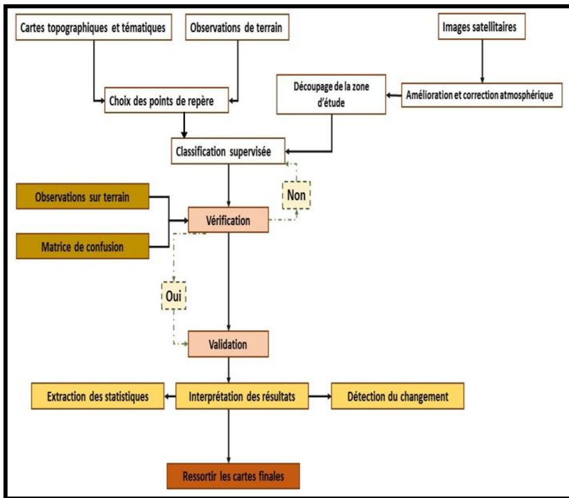
Figure 44 : Diagramme méthodologique du suivi des changements spatiotemporels de l'occupation du sol.
