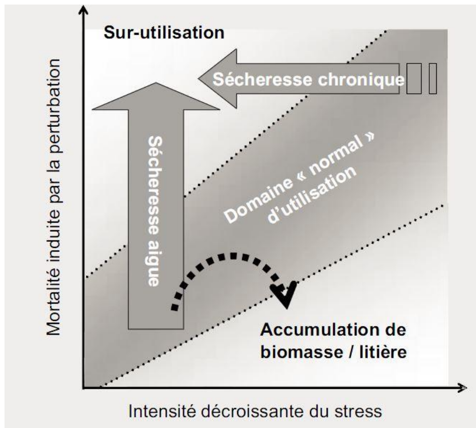
Figure 43: Effet de la sécheresse sur les systèmes pastoraux (intensité et fréquence) (Alard et Balent, 2007)
