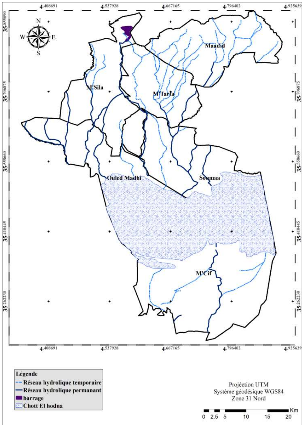
Figure 10 : Réseau hydrographique (extraite du modèle numérique du terrain MNT)
