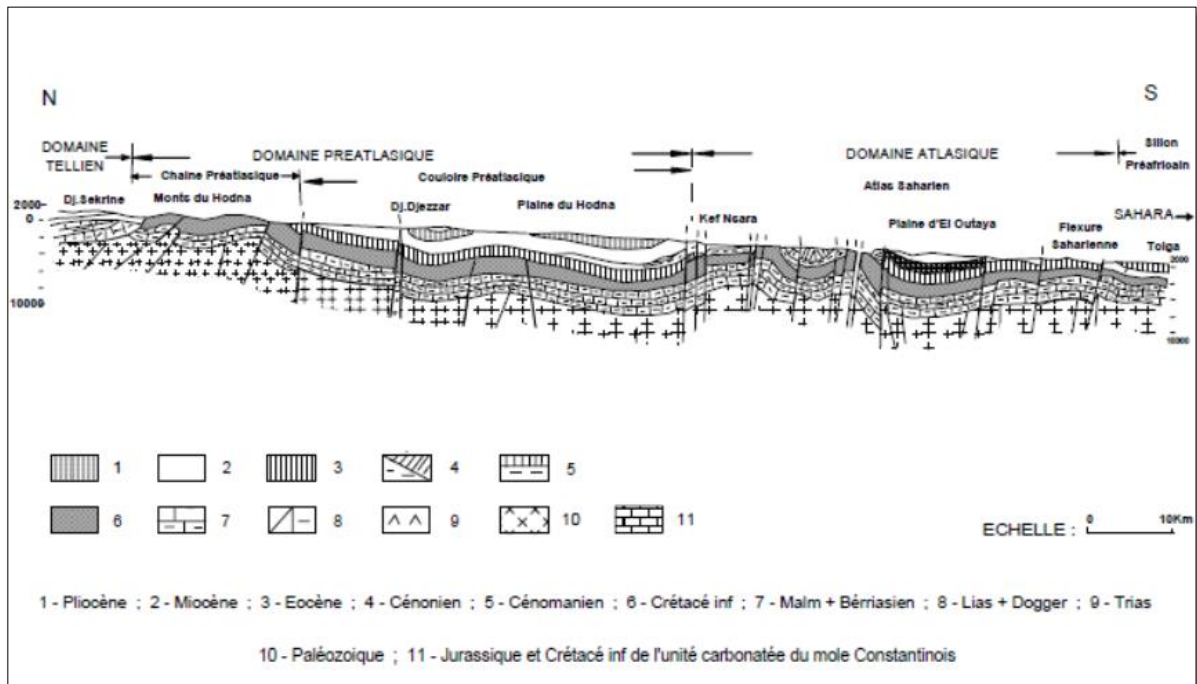
Figure 7 : Coupe schématique de la région du Hodna (F.A.O 1968)
