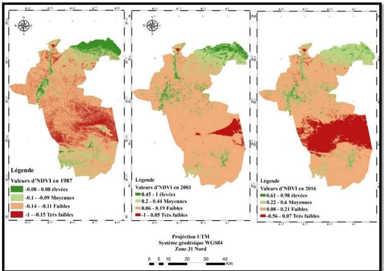
Figure 50 : Carte de l'indice NDVI des années 1987, 2003, 2016.
