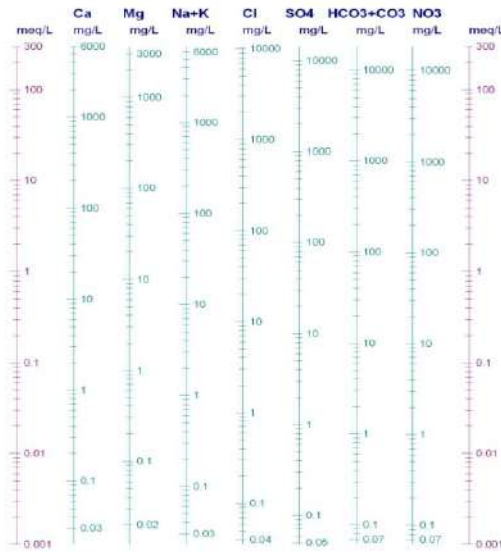
Figure 49 : Diagramme de Schoeller-Berkalof
