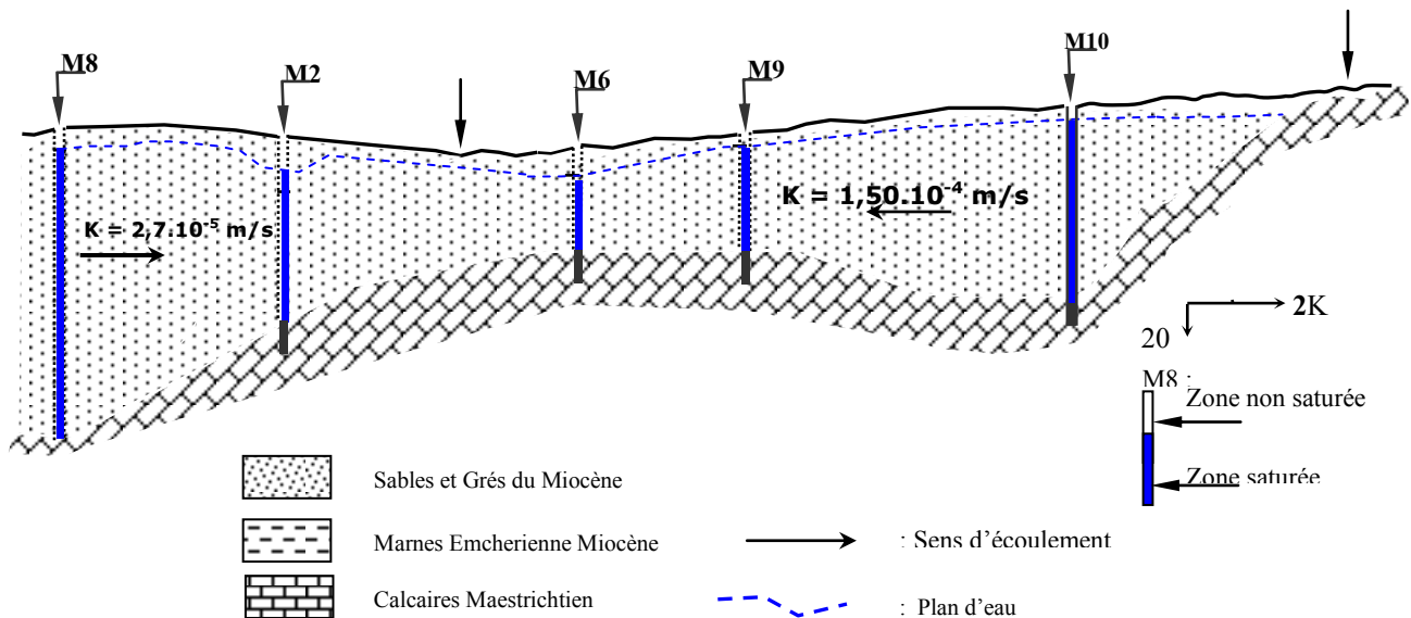
Figure 22 : Coupe hydrogéologique à travers la plaine d'El Ma El Abiod Rouabhia et al. 2009
