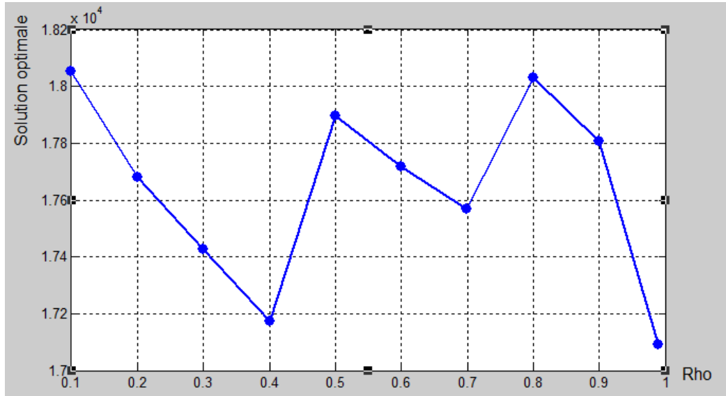
Fig.III.18. Détermination du paramètre \rho cas : la demande est générale
