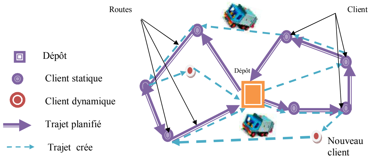
Fig. I.6. Création d'une nouvelle route
