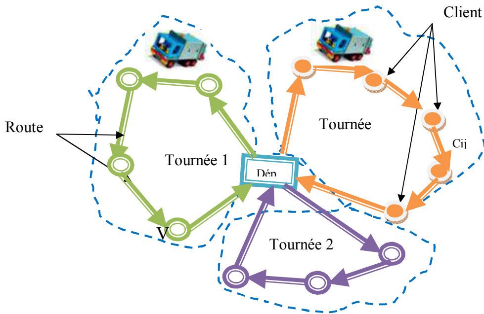
Fig. I.2 Présentation graphique du problème de tournées de véhicules VRP
