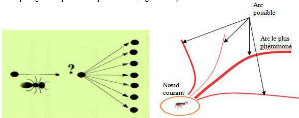
Fig. II. 8. a : Sélection du chemin par la fourmi de façon aléatoire
