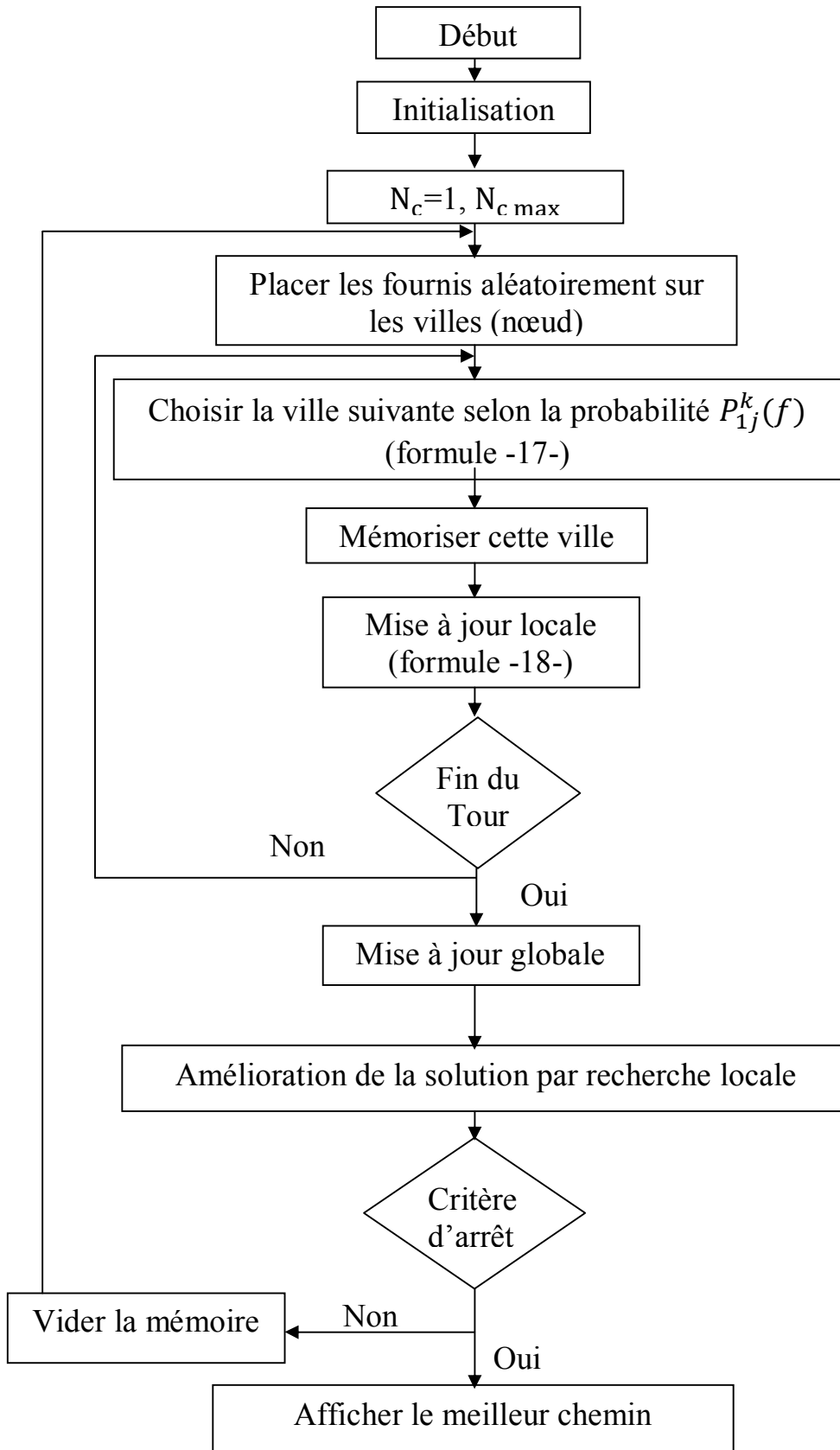
Fig. II.10 Organigramme de l'algorithme de base d'ACO
