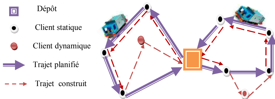
Fig. I.5 Construction d'une nouvelle route
