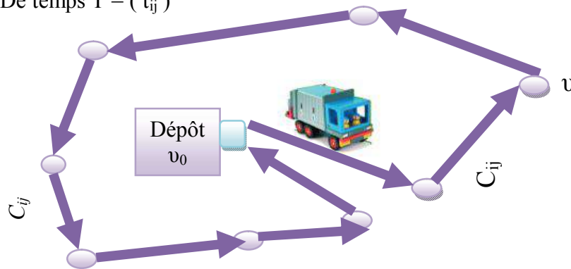
Fig. I.1 Présentation graphique du problème de voyageur de commerce TSP
