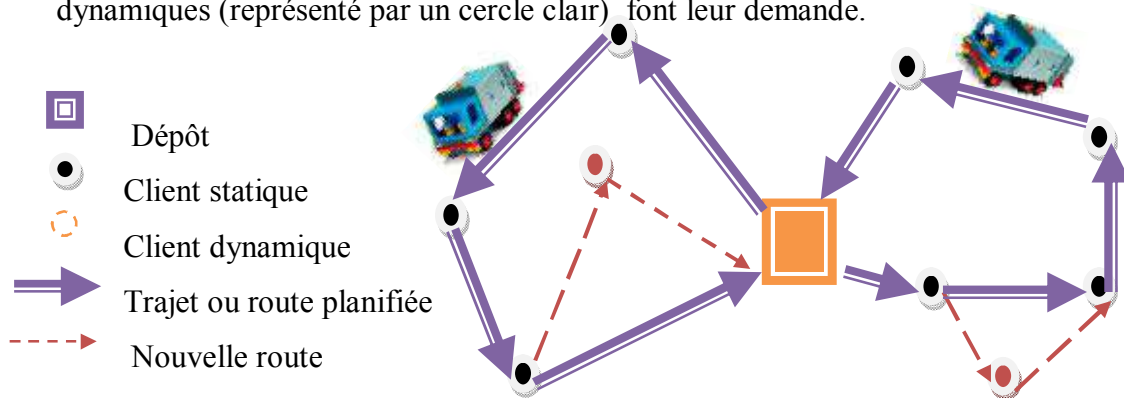
Fig. I.4 problème VRP statique et dynamique [GON 06]
