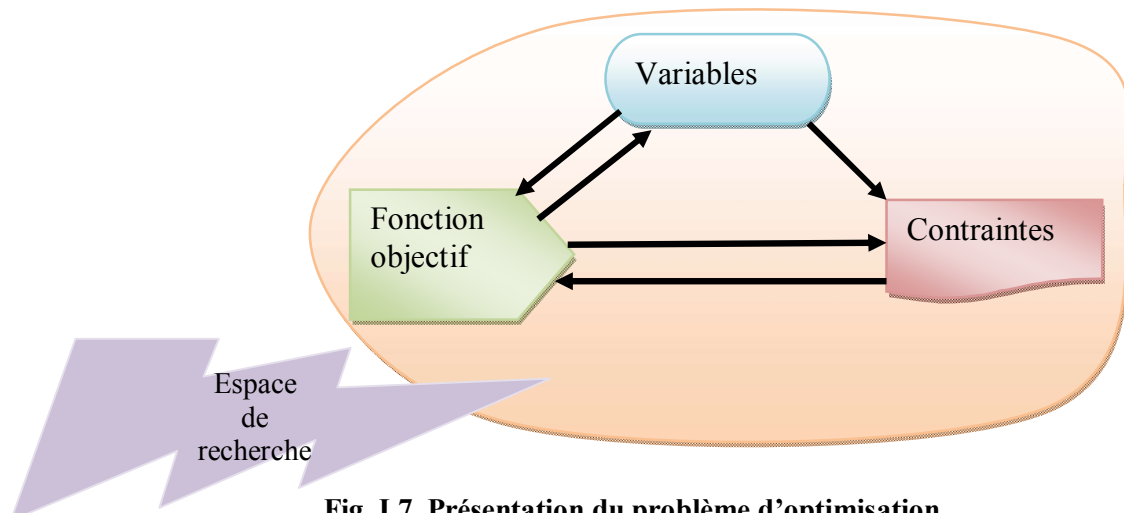
Fig. I.7 Présentation du problème d'optimisation
