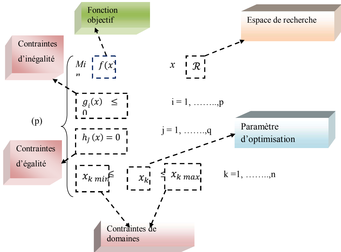
Fig. I.8: Présentation mathématique d'un problème d'optimisation multi objectif [SAA07]
