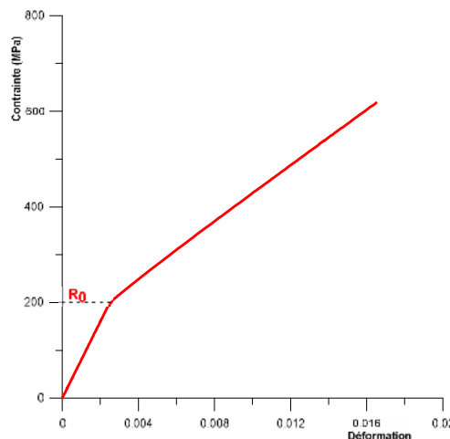
Fig. I.9 : Représentation de la loi de comportement élastoplastique avec écrouissage isotrope.
