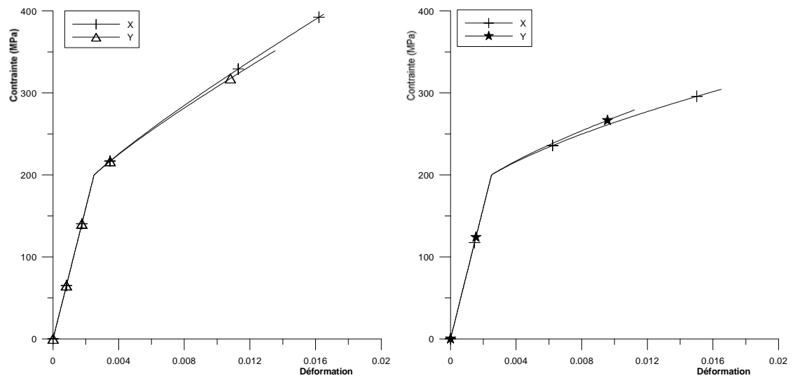
Fig. IV.15: Nature du comportement apparent dans la direction de sollicitation Y, courbes de traction, fraction volumique: P (0.1 – 0.6).
