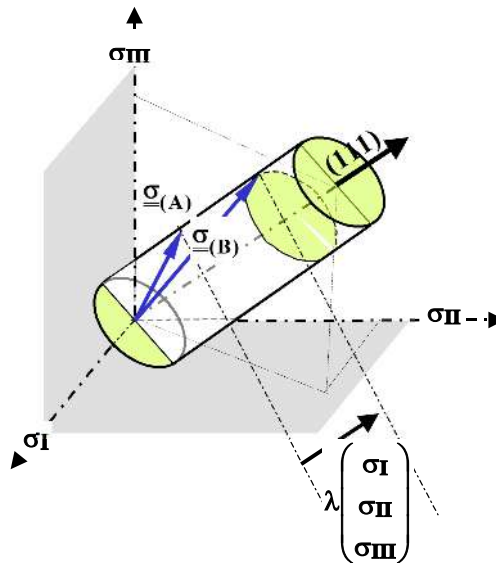
Fig. I.4 : Surface de von Mises dans l'espace des contraintes principales avec deux états de contraintes satisfaisant \bar{\sigma} = R_e .
