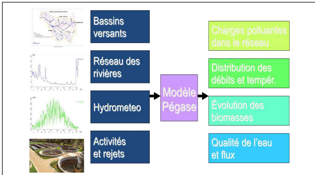
Figure II.7. Principe de fonctionnement général de Pégase (Aquapôle, ULg)
