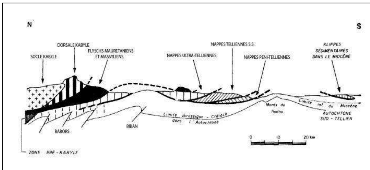
Figure III.12. Rapports structuraux entre les différentes unités de la chaîne des Maghrébides
