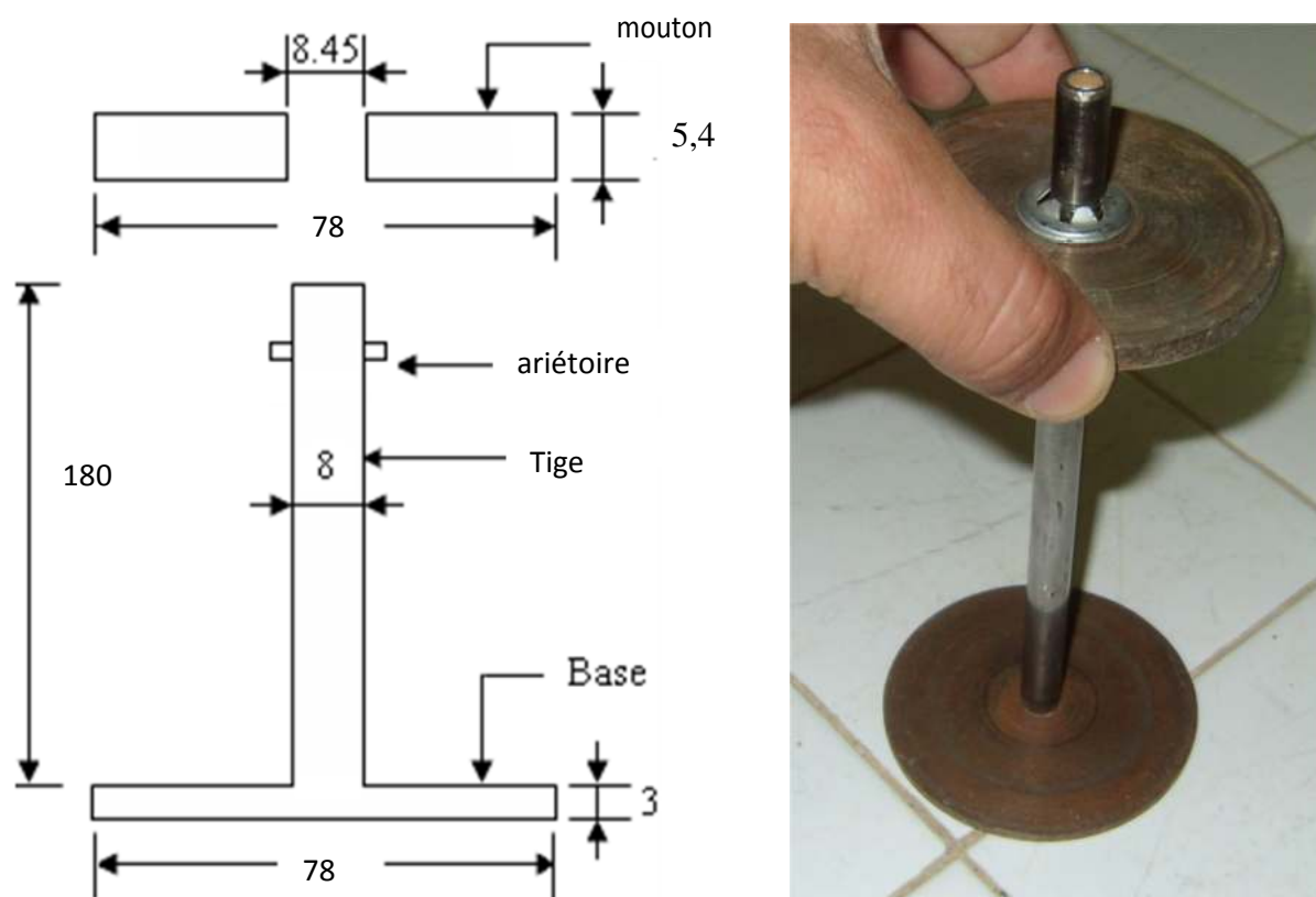
Figure.2.7. L'appareillage de compactage d'échantillon.
