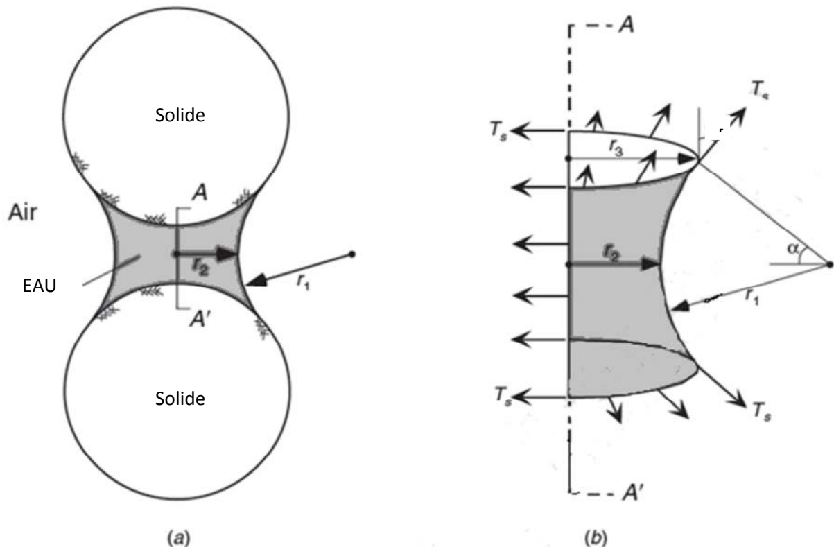
Figure.1.12. La géométrie idéalisée d'interface de l'air-eau dans les sols non saturés (Ning et William 2004); a)Ménisque de l'eau entre deux particules sphériques de sol ; b) Le diagramme de libre-corps pour le ménisque de l'eau.
