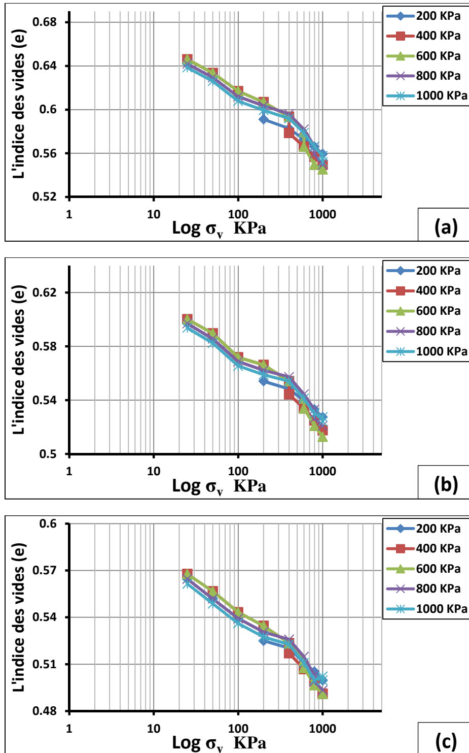
Figure.3.8. Les courbes obtenus à partir les essais œdométriques simples effectués sur le sol S1 à teneur en eau initiale ( w=6\% ). (a) E_c = 20 coups ; (b) E_c = 40 coups ; (c) E_c = 60 coups.
