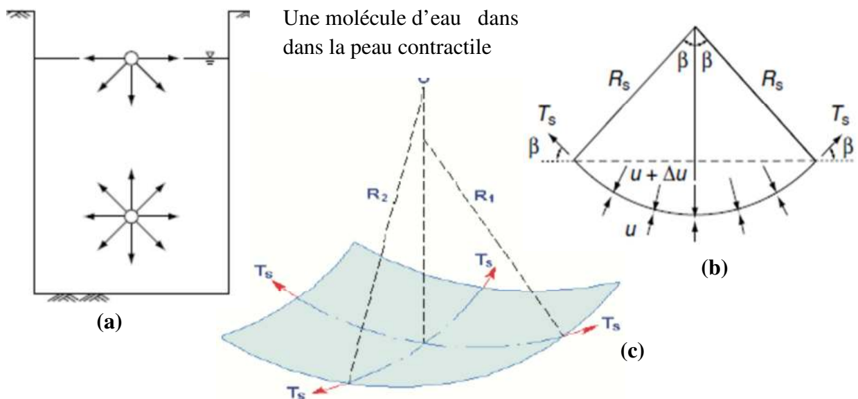
Figure.1.11. La tension superficielle à l'interface de l'air-eau (Fredlund et Rahardjo 1993); a) les forces intermoléculaire b) les pressions agissant sur incurvé surface bidimensionnel ; c) la tension superficielle à la peau contractile en (3D).
