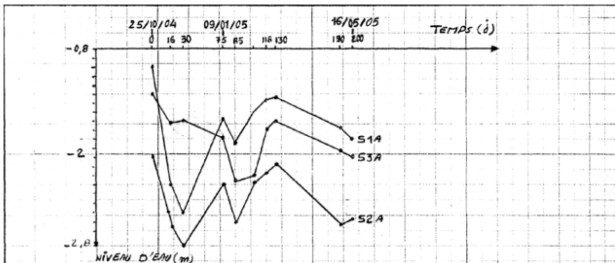
Fig.V.9 : Evolution du niveau d'eau dans les sondages (Selon les données de l'OPGI de Mila, 2006).
