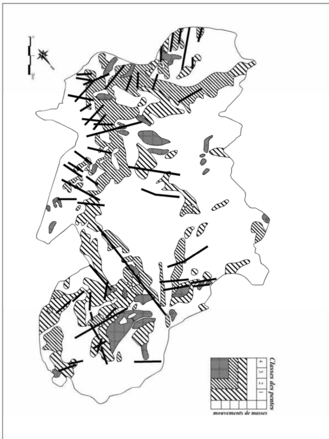
Fig. VI.5 : carte synthétique N° II : mouvements de masse selon la pente.
