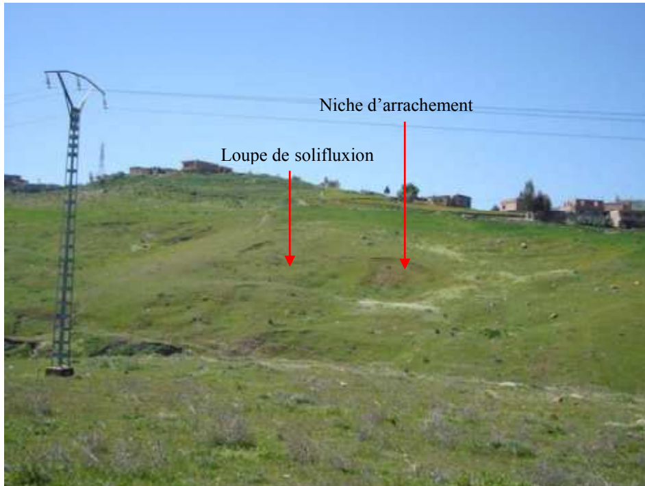
Fac-similé IV.1 : loupes de solifluxion et foîrage en paquet dans un versant.
