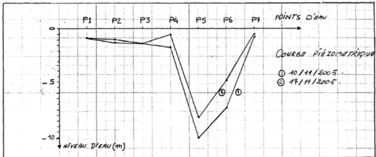
Fig.V.8 : Evolution du niveau d'eau dans les piézomètres (Selon les données de l'OPGI de Mila, 2006).
