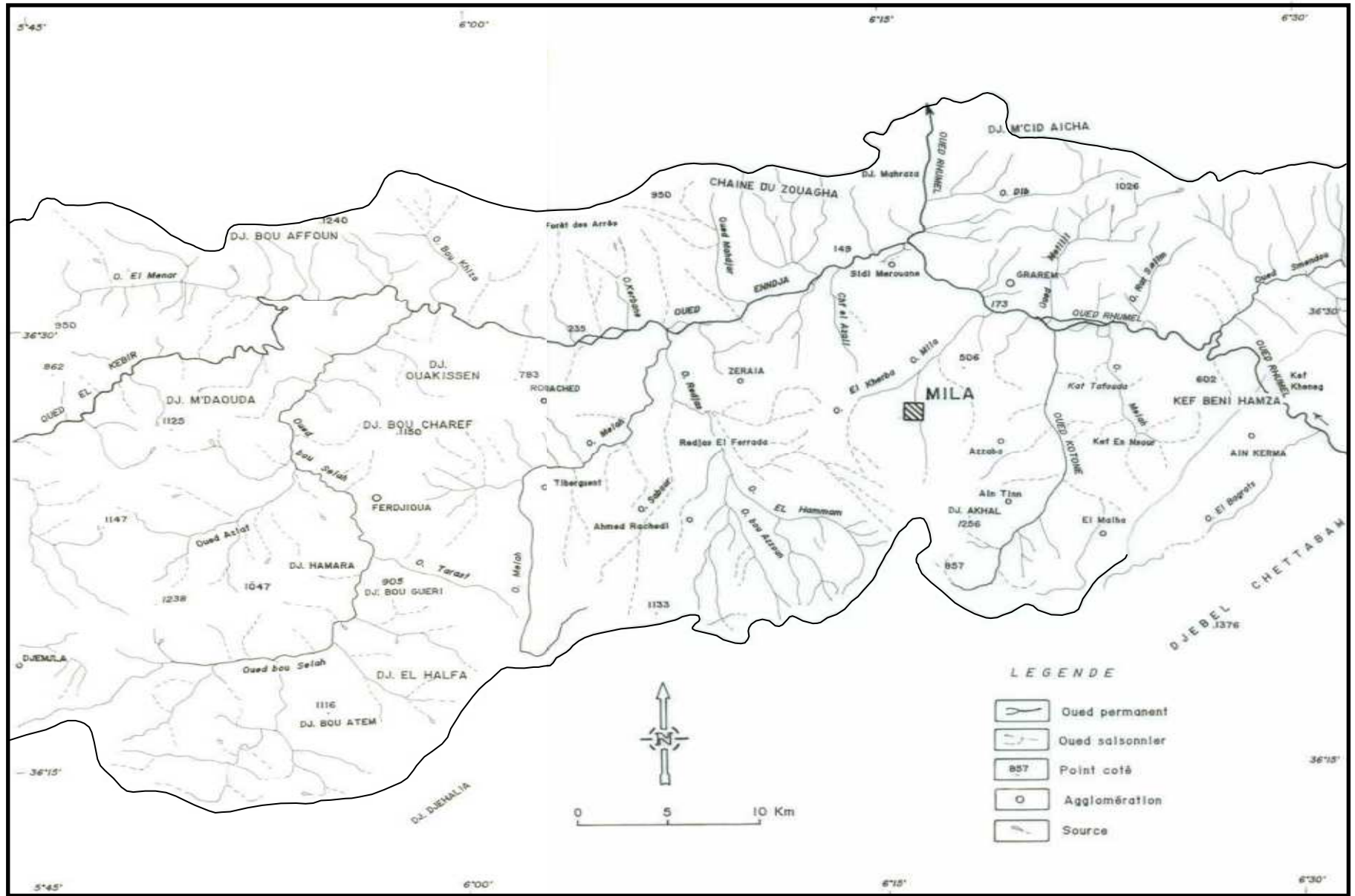
Fig.I.2 : Réseau hydrographique du bassin de Mila.
