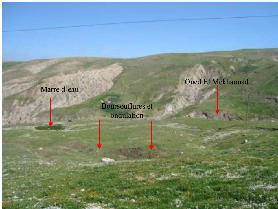
Fas-similé IV.3 : Boursouflures et marre d'eau près au pied d'Oued Mekhaoued.
