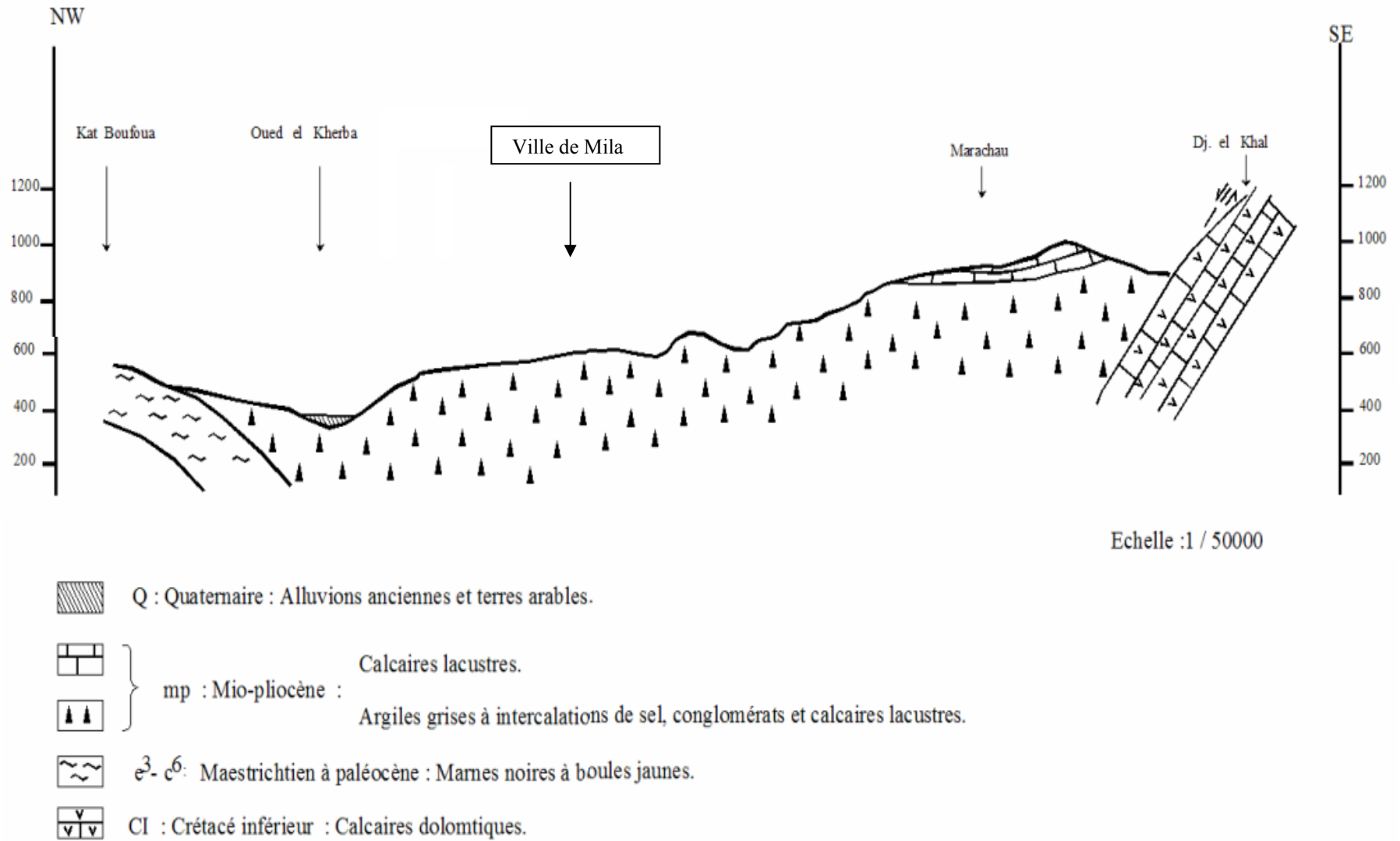
Fig I.8 : Coupe géologique passant par la ville de Mila (J.M. Vila, 1977).
