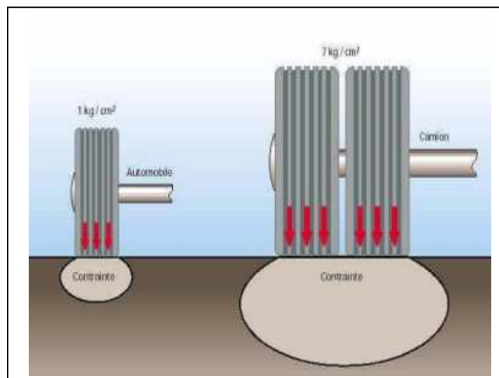
Fig.1.9 : Schéma de principe illustrant les agressivités respectives vis-à-vis de la chaussée d'un véhicule léger et d'un poids lourd
