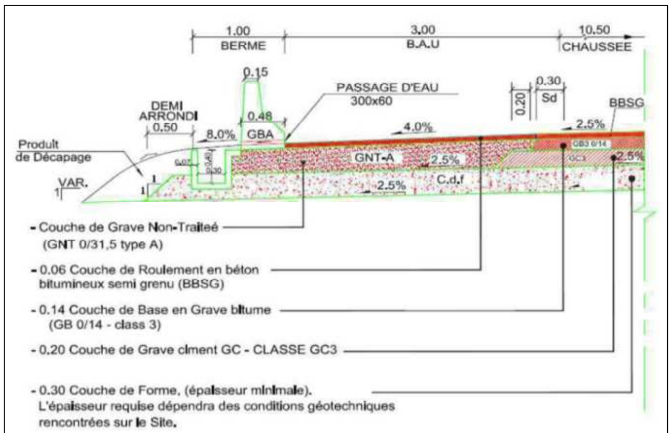
Fig.1.14 : Structure type de la chaussée et accotement
