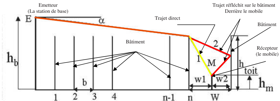
Figure II.13 : Profil synthétique du modèle COST 231.
