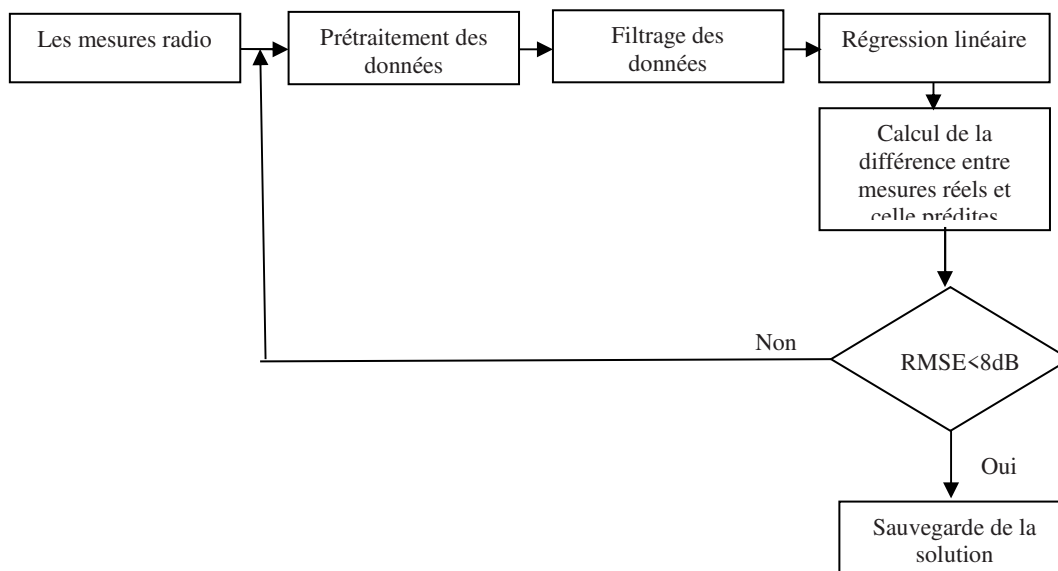
Figure IV.11 : Organigramme de l'algorithme d'optimisation.
