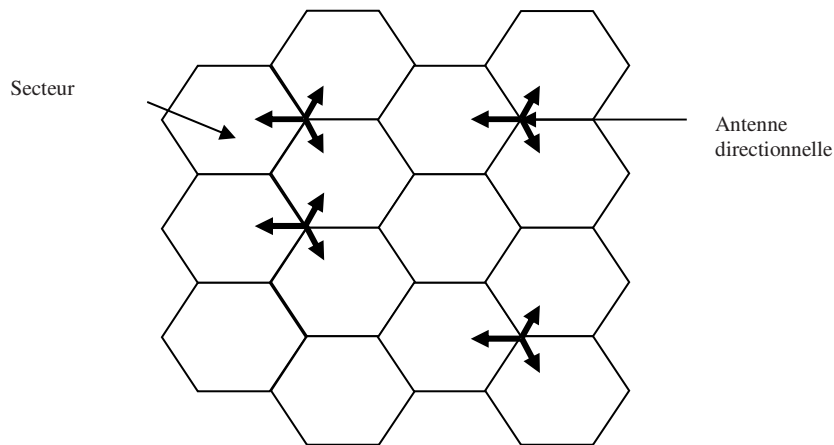
Figure I.29: Topologie d'un réseau cellulaire trisectorisé à structure hexagonale.
