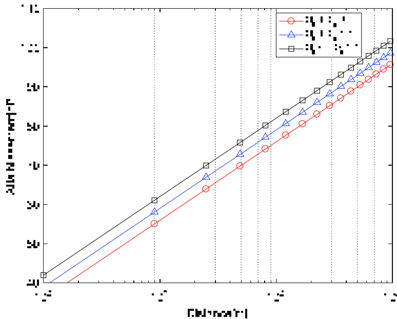
Figure III.12 : Modèle d'affaiblissement en espace libre.
