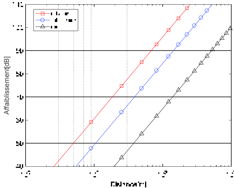
Figure III.16 : Affaiblissement de parcours pour le modèle Okumura- Hata.
